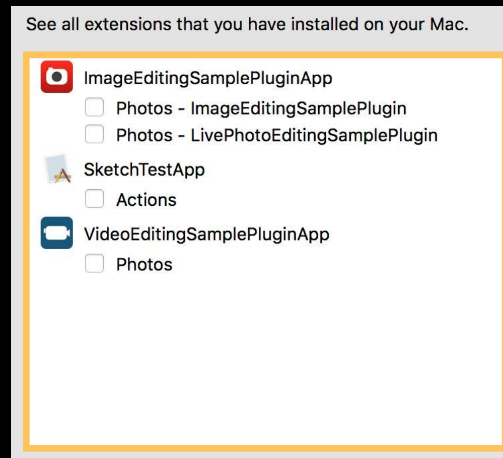
NSTableView
