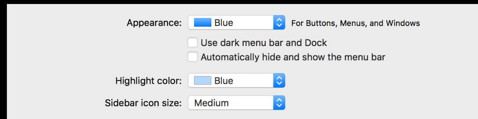
NSGridView
