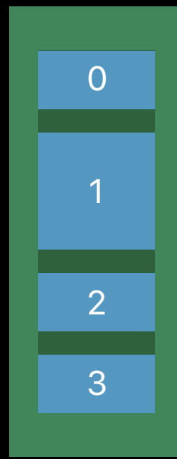
NSStackView
