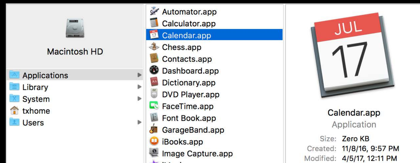
NSBrowser
