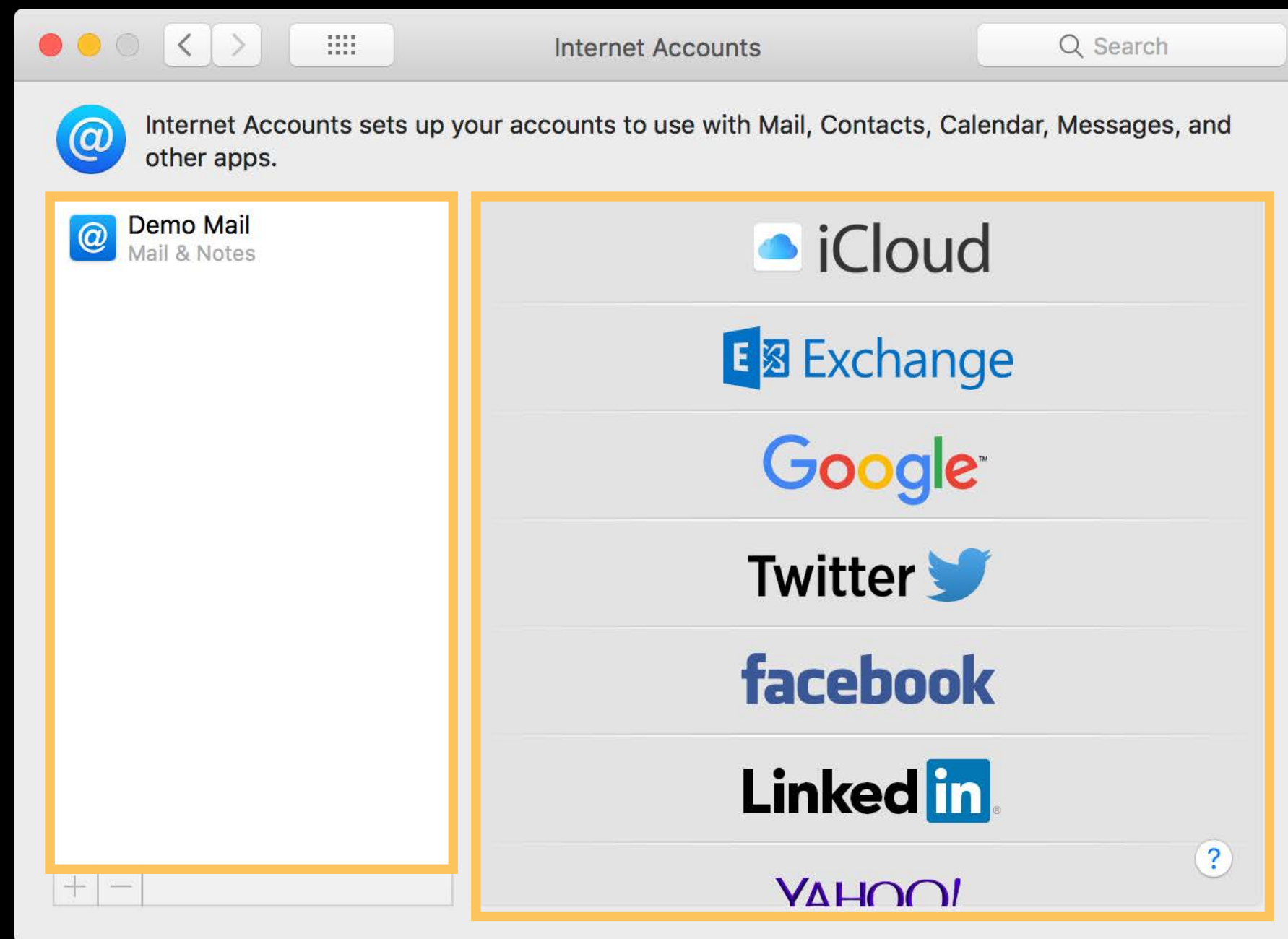
NSTableView
