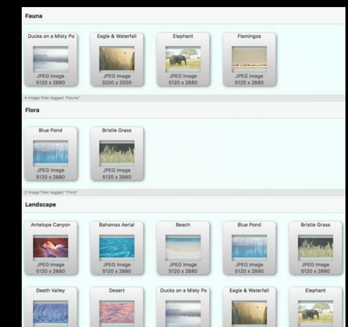
NSCollectionView
