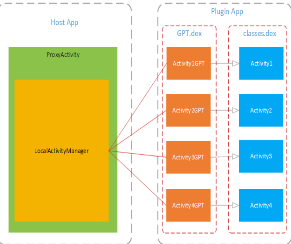
3代插件系统-GPT
