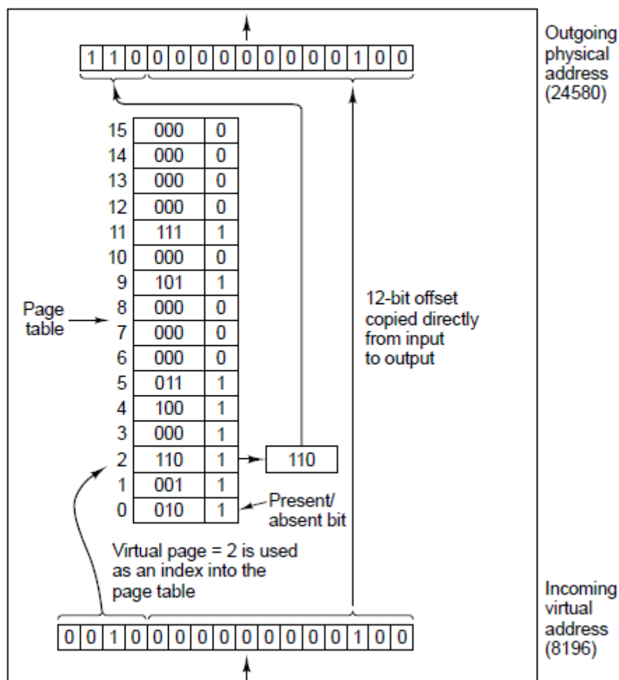
图4-9 在16个4K页的情况下MMU的内部操作。
