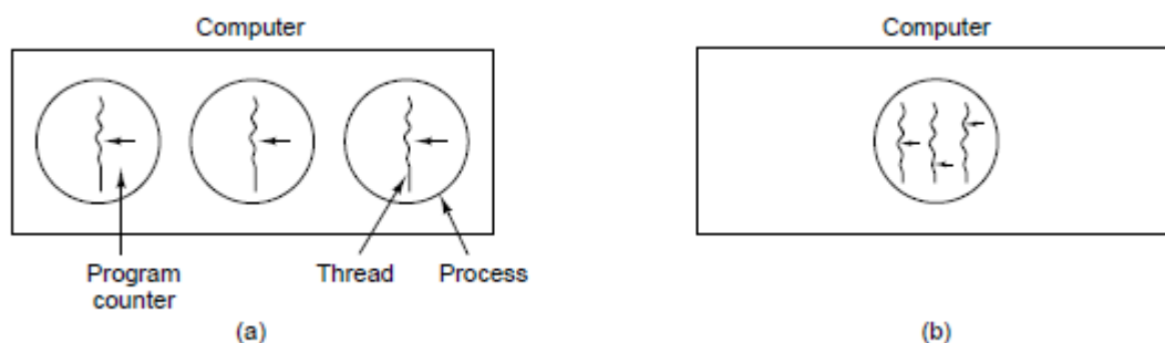
图2-6 (a) 三个进程各有一个线程。(b) 一个进程有三个线程。
