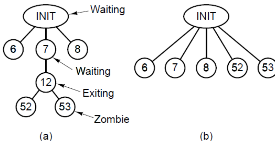
图4-43 (a) 进程12要结束时的情况。(b) 进程12结束以后的情况。
