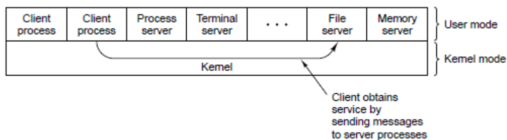
图 1-20 客户/服务器模型。
