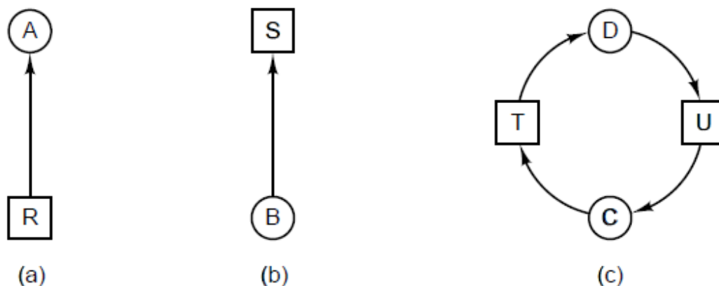
图 3-7 资源分配图。(a) 占用一个资源 (b) 请求一个资源 (c) 死锁
