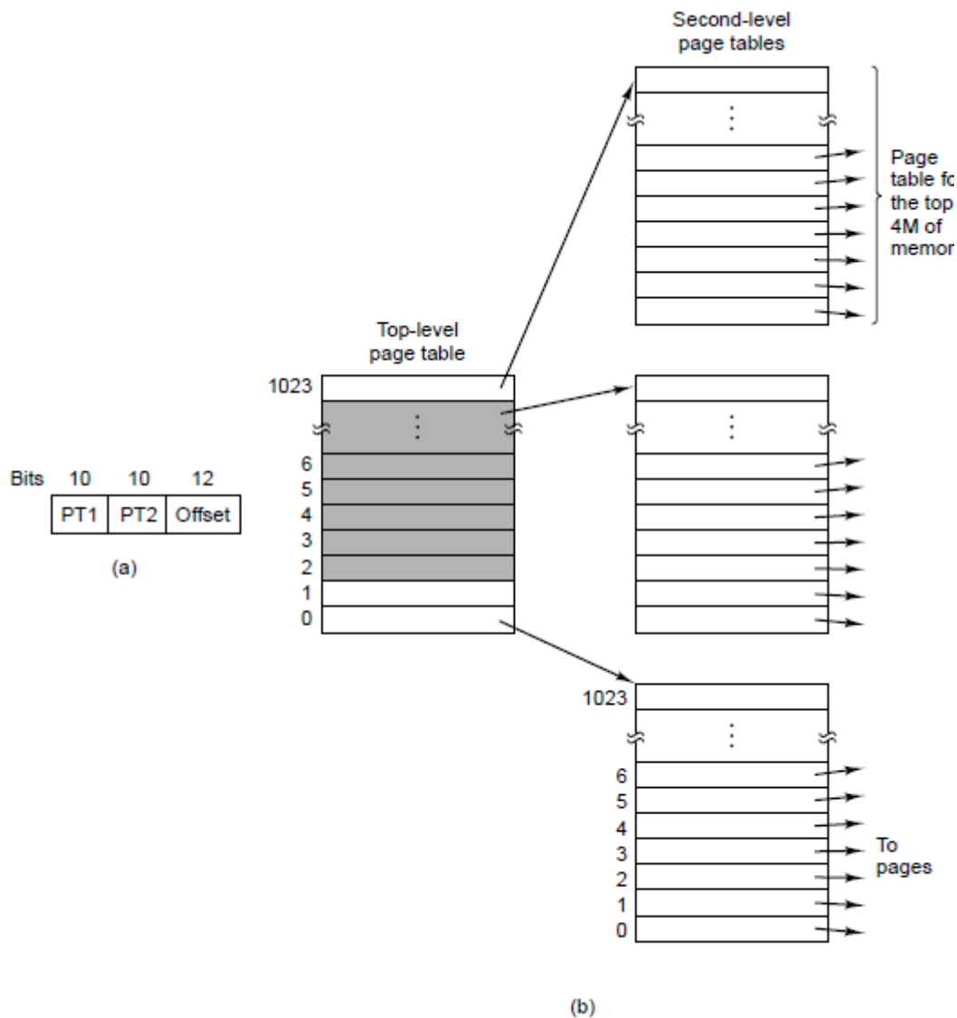
图4-10 (a)一个有两个页表域的32位地址。(b)二级页表。
