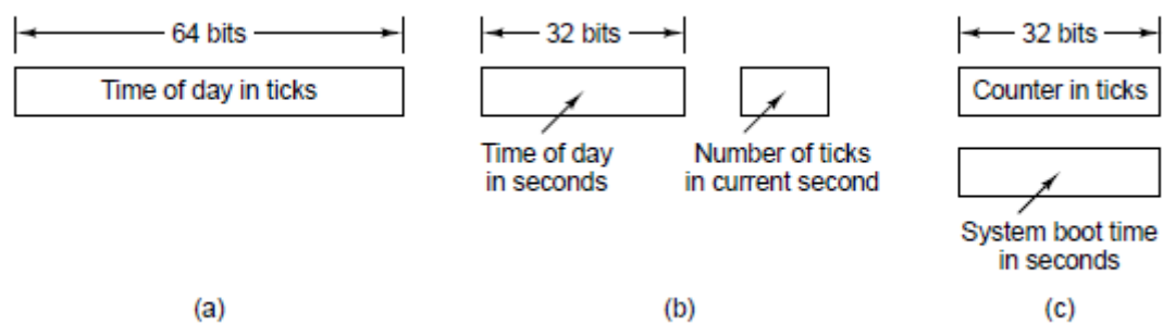
图 3-24 维护每天时间的三种方法。
