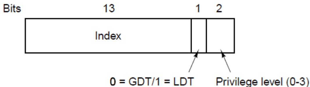
图4-27 一个奔腾的选择符。
