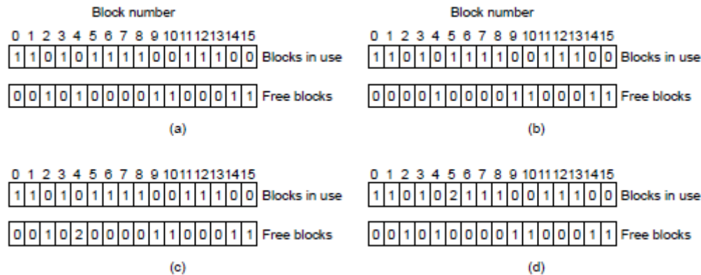
图5-18 文件系统状态：(a)一致 (b)块丢失 (c)空闲表中有重复块 (d)重复数据块
