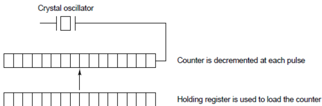
图 3-23 可编程时钟。
