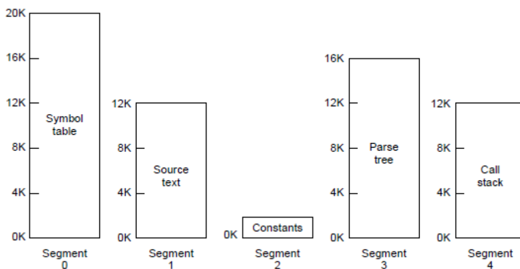
图4-20 分段的内存允许各个表独立地增长或缩减。
