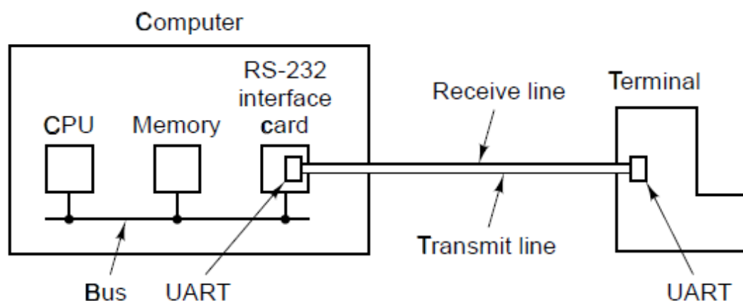
图 3-30 一个 RS-232 终端通过一条一次传输一位的通讯线路和计算机通讯。计算机和终端完全独立。
