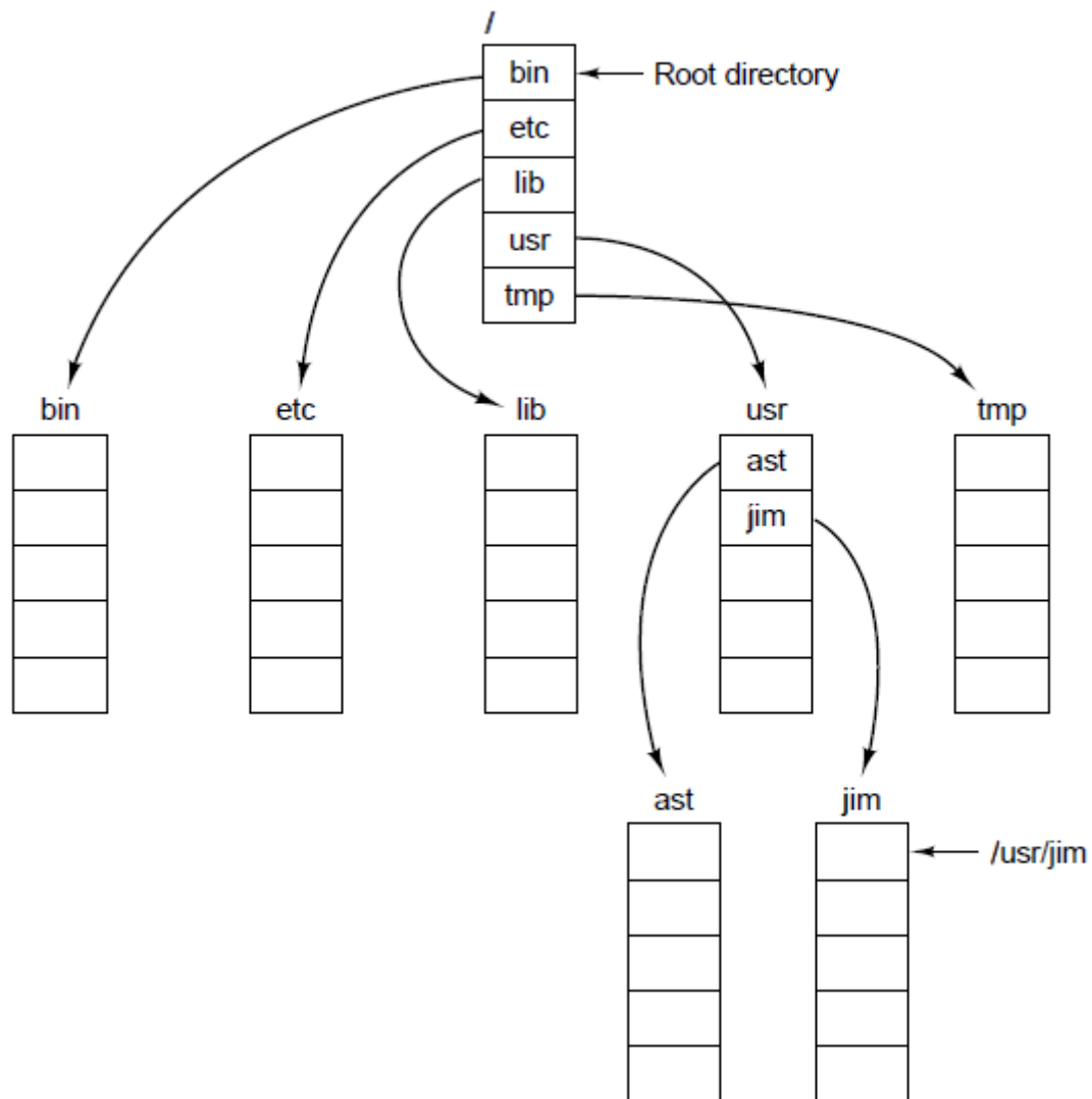
图5-7 一棵UNIX目录树。
