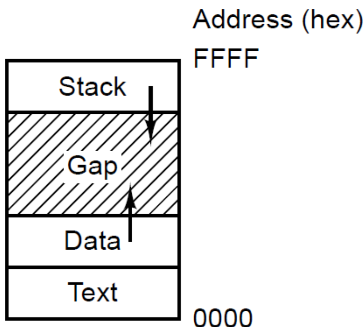
图 1-11 进程有三个段：正文段、数据段和堆栈段。在本例中，所有三个段在同一个地址空间中，但是也支持分离的指令空间和数据空间。
