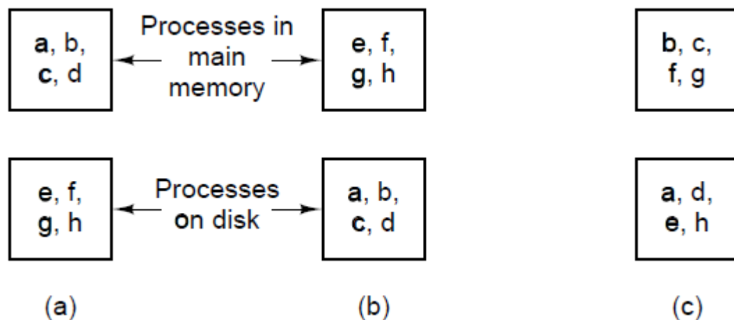
图2-25 两级调度程序必须将进程在磁盘和内存间来回移动，并从驻留在内存的进程中进行选择。
