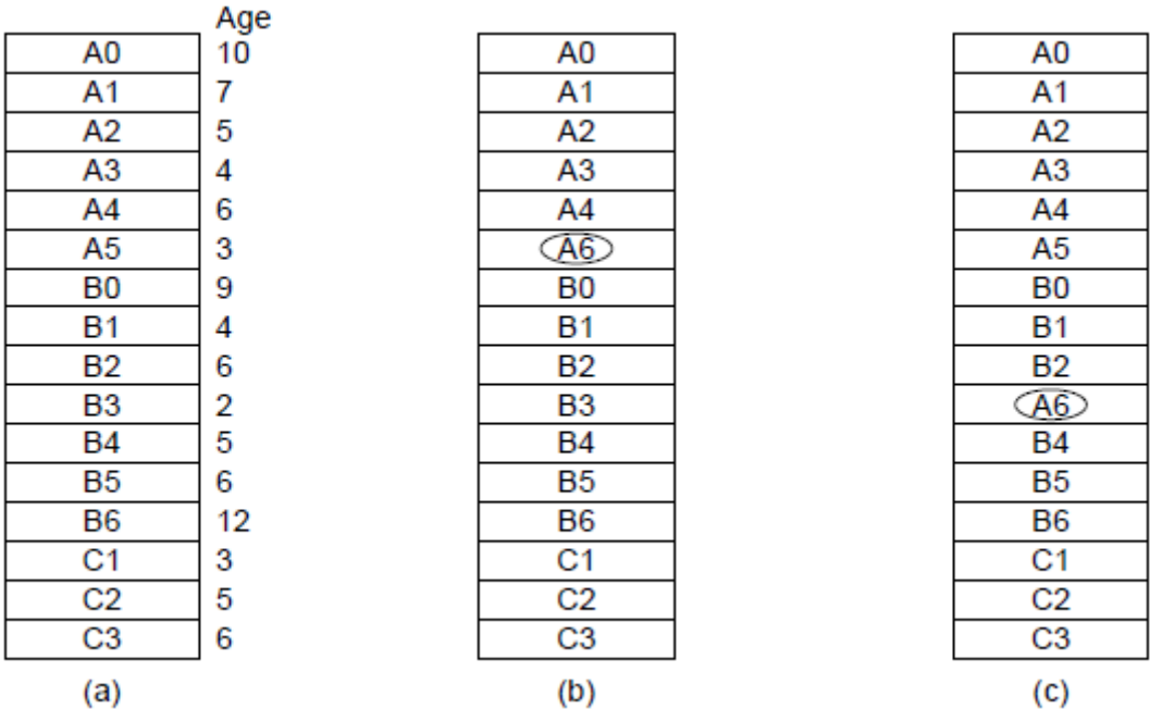
图4-17 局部与全局替换算法。(a)原先配置。(b)局部页面替换。(c)全局页面替换。
