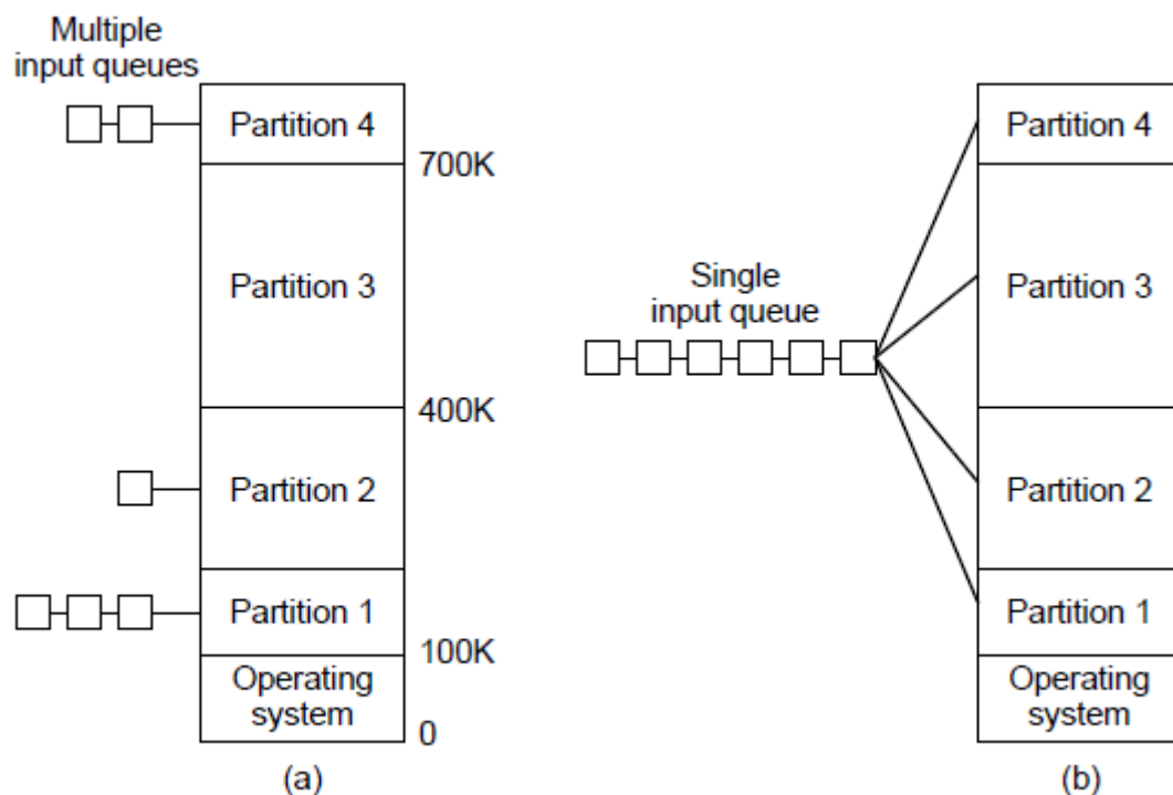
图4-2 (a)各分区具有独立输入队列固定内存分区。(b)仅有单个输入队列的固定内存分区。
