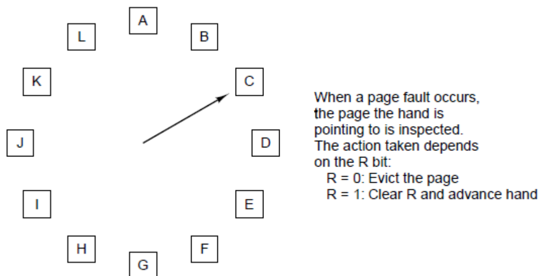
图4-14 时钟页面替换算法。
