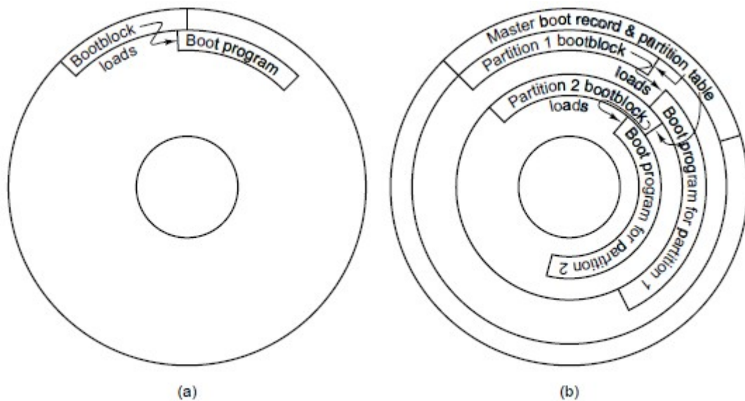
图 2-31 引导使用的磁盘结构。(a) 未分区的磁盘，第一扇区就是引导块。
