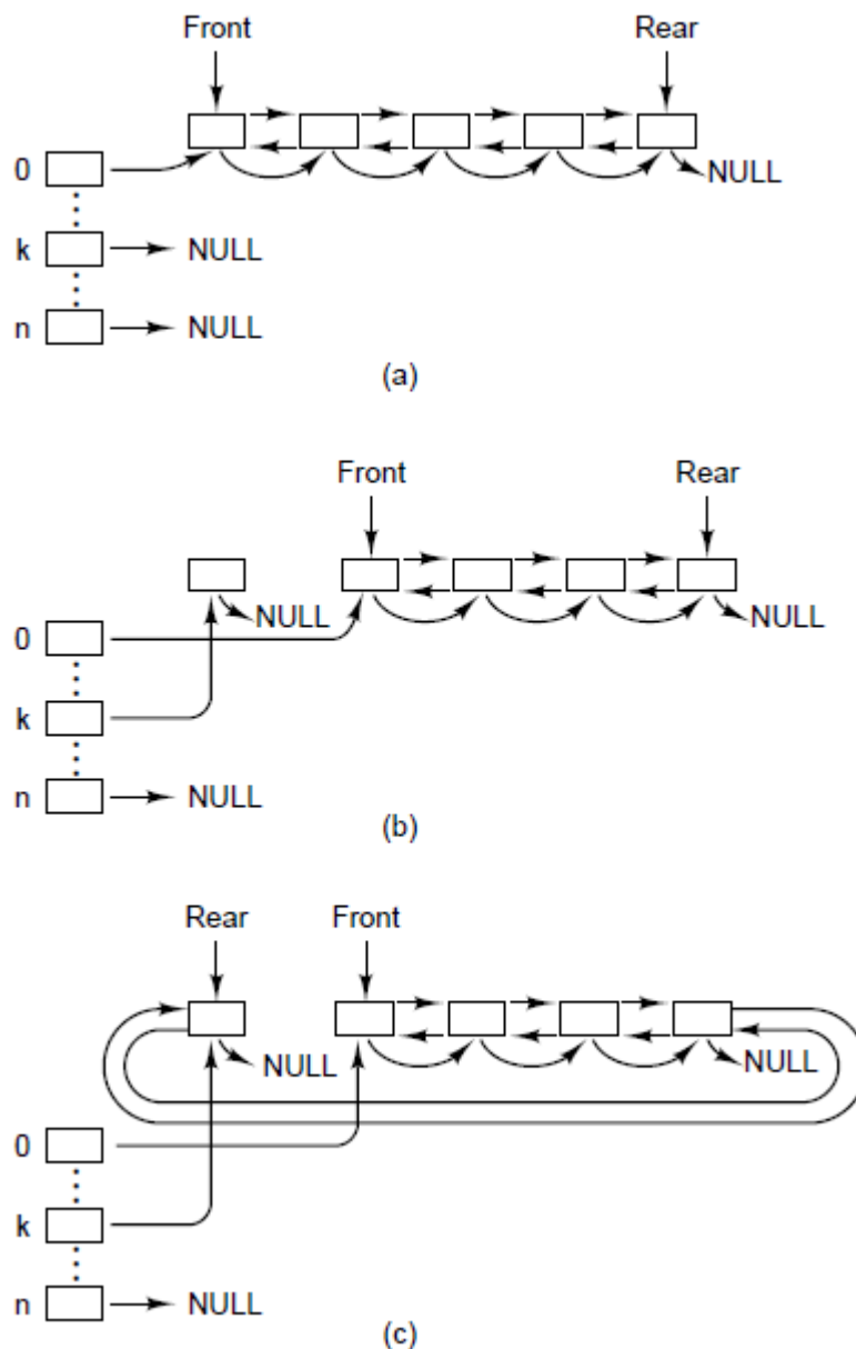
图5-38 块高速缓存的初始化。(a)在使用任何缓冲区之前。(b)在请求一块后。 (c)在该块被释放后。
