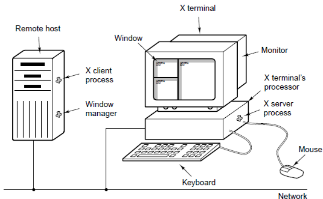
图 3-31 M.I.T X 窗口系统中的客户和服务。
