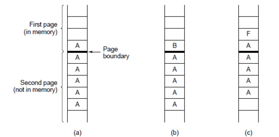
图5-20 TENEX口令问题。
