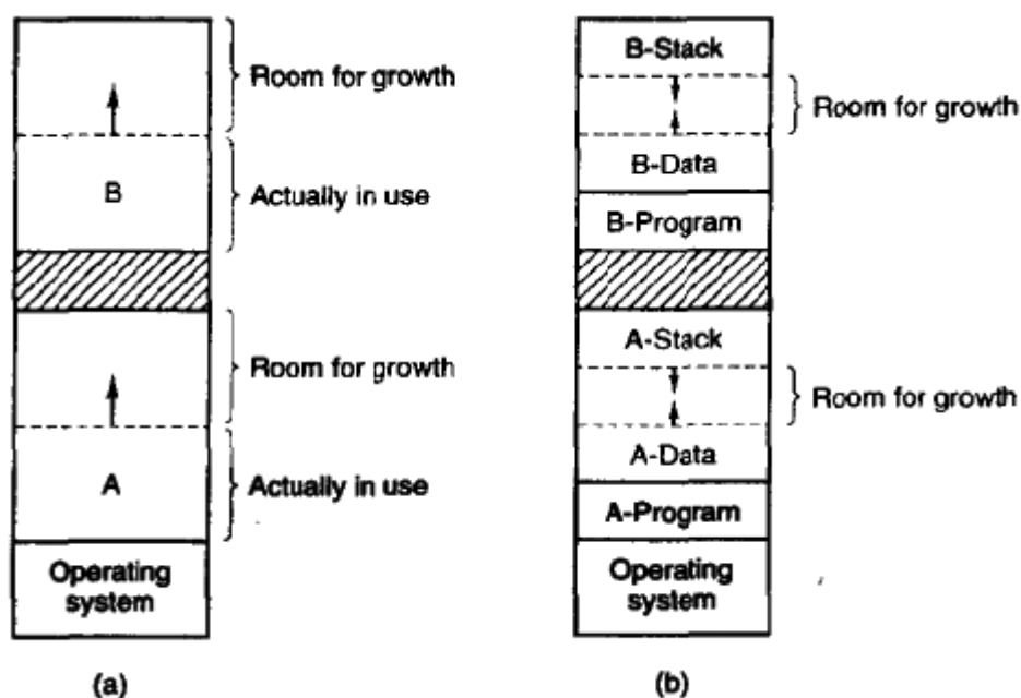
图4-4 (a)为能够增长的数据段预留空间。(b)为能够增长的数据段和堆栈段预留空间。
