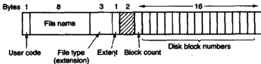
图5-11 目录项中包含每个文件的磁盘块号。
