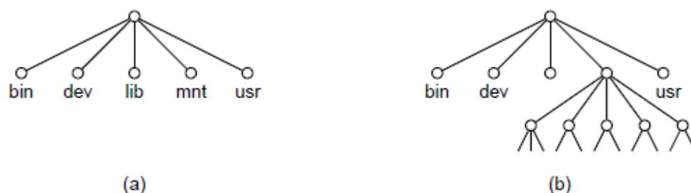
图 1-15 (a) 安装前的文件系统。 (b) 安装后的文件系统。
