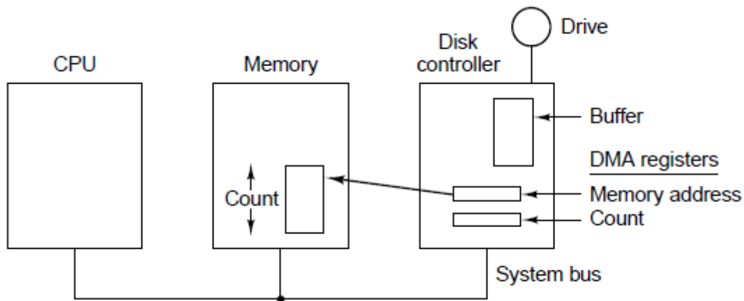
图 3-3 一次DMA传输完全由控制器完成。
