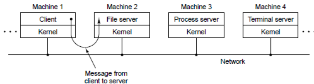
图 1-21 在一个分布式系统中的客户/服务器模型。
