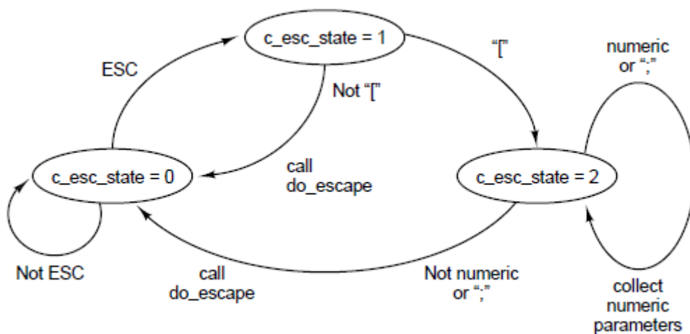
图 3-48 处理转义序列的有限状态机。
