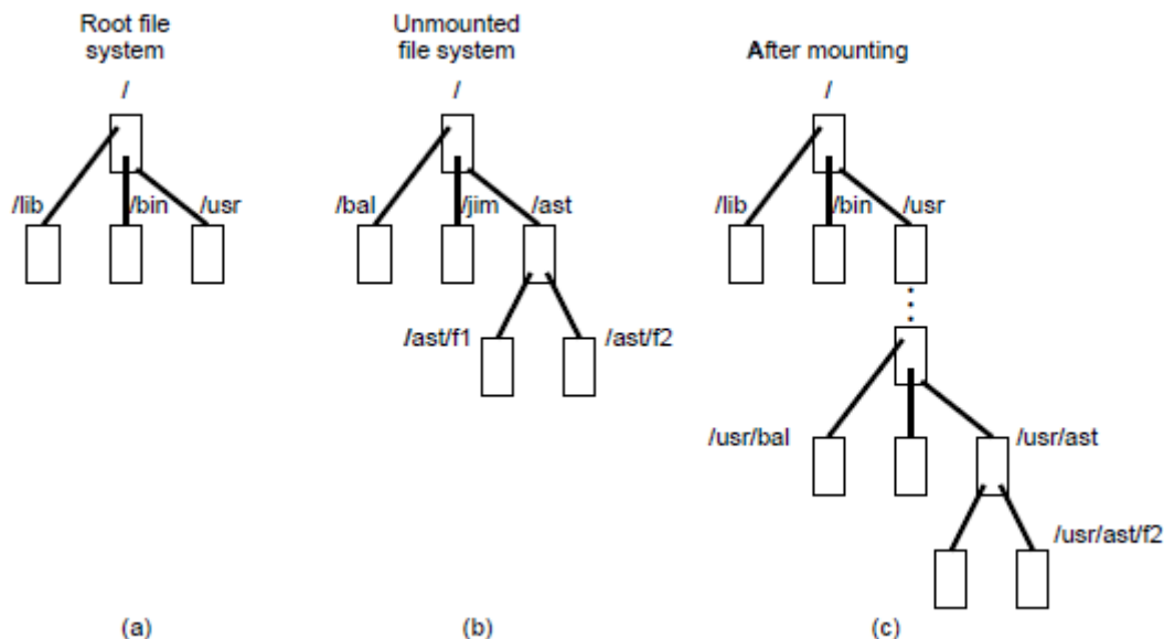
图5-32 (a)根文件系统。(b)未被安装的文件系统。(c) (b)的文件系统安装到目录/usr后的效果。
