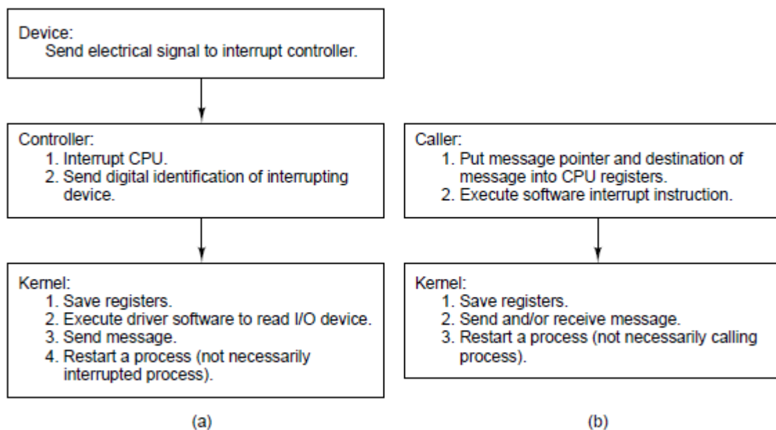
图 2-34 (a)硬件中断的处理过程。(b)系统调用处理过程。
