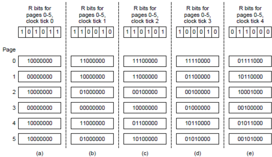
图4-16 用软件模拟LRU的老化算法。图中所示是6个页面在5个时钟周期的情况，5个时钟周期分别由(a)–(e)表示。
