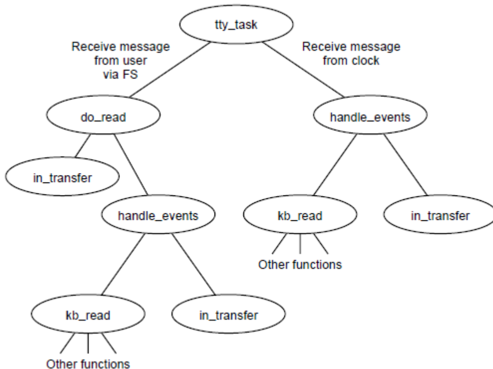
图 3-38 终端驱动程序的输入处理。树的左分枝表示处理一个读字符请求。右分枝表示向驱动程序发送了一条“字符已被输入”消息。
