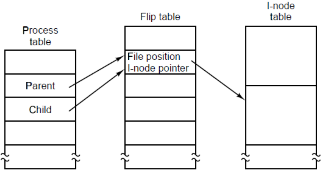
图5-33 父进程与子进程共享文件位置。
