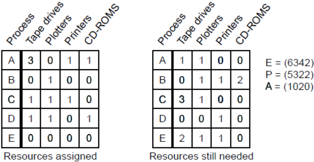
图 3-13 多种资源的银行家算法。
