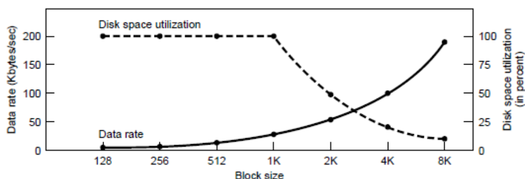
图5-15 实线(左边标度)给出磁盘数据率，虚线(右边标度)给出磁盘空间效率，所有文件均为1K。
