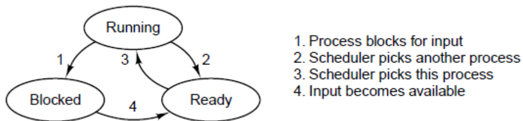
图2-2 一个进程可处于运行态、阻塞态、就绪态。图中示出各状态之间的转换。
