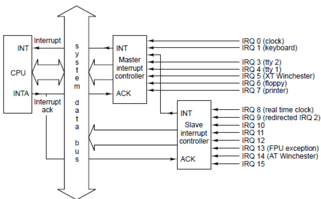
图2-33 一台32位Intel PC上的中断处理硬件。
