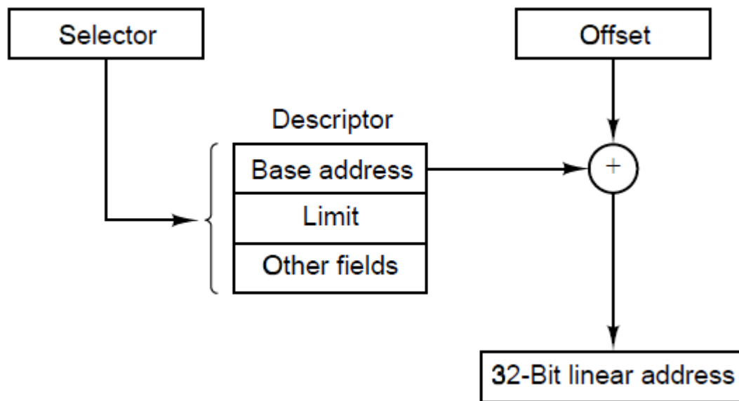
图4-29 （选择符、偏移）到线形地址的转换。
