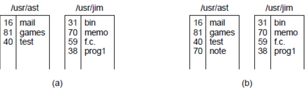
图 1-14 (a)将/usr/jim/memo链接到ast的目录之前的两个目录。
