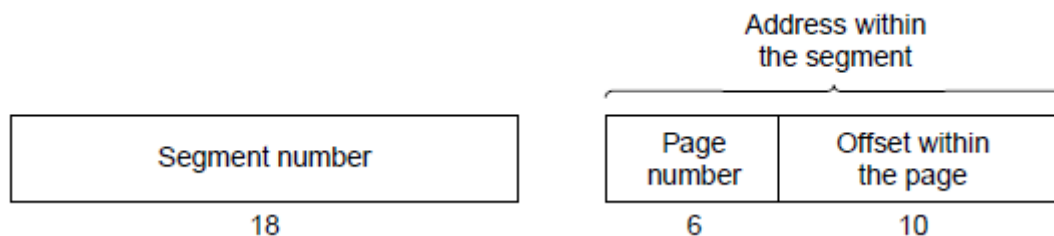
图4-24 34位的MULTICS虚地址。
