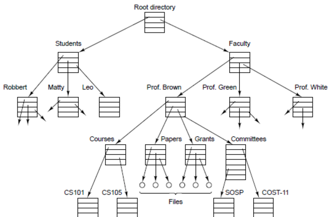
图 1-6 大学里一个系的文件系统。
