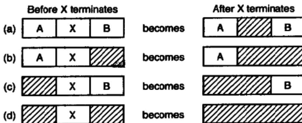
图4-6 进程X终止时四种与邻居合并的方式。
