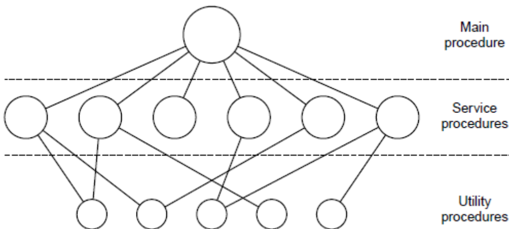
图 1-17 整体式操作系统的简单结构模型。
