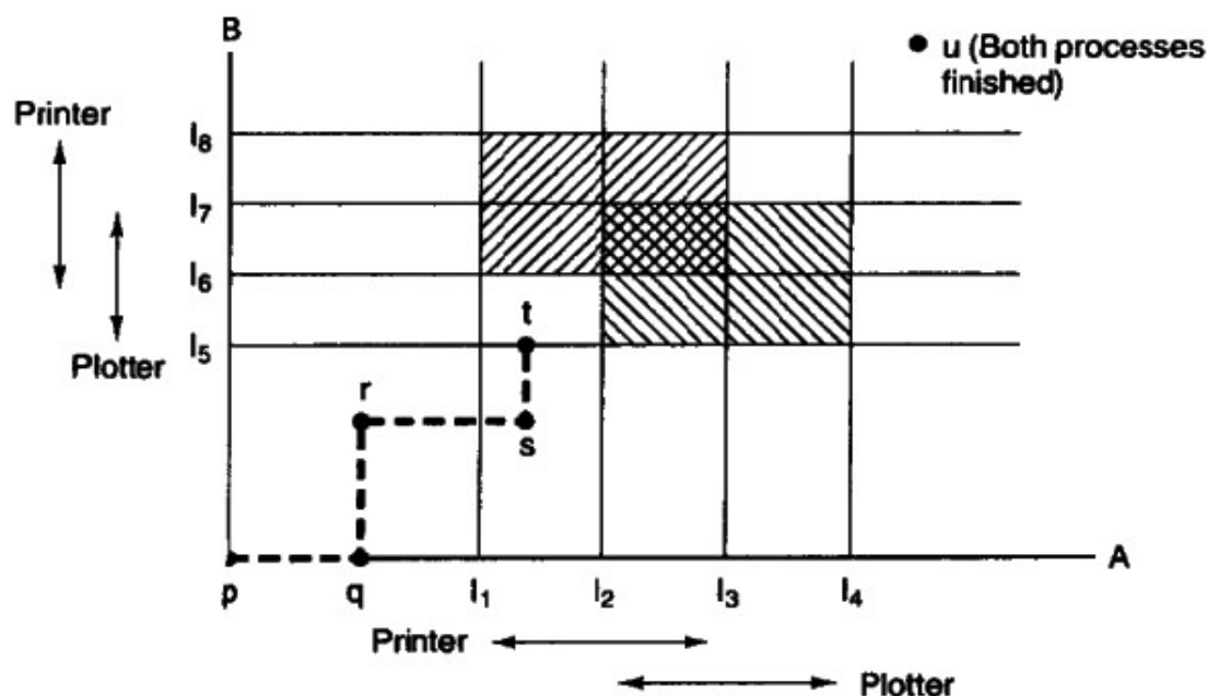
图 3-12 两个进程的资源轨迹图。
