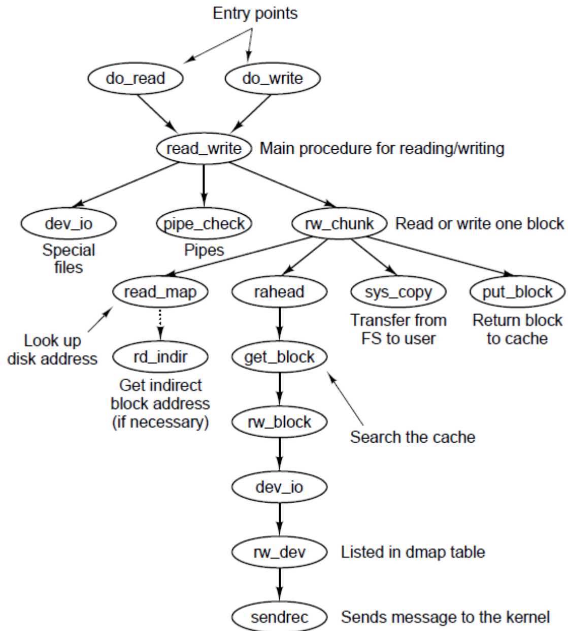
图5-40 用于读文件的一些过程。
