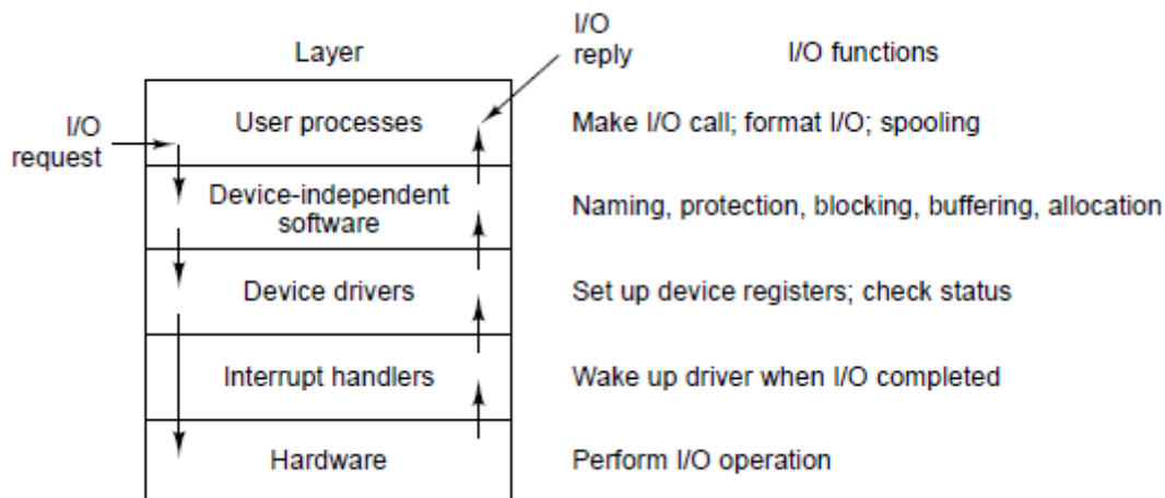
图 3-6 I/O系统的层次结构及各层的主要功能。
