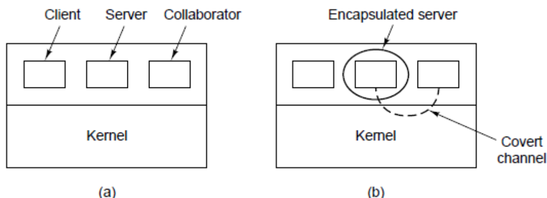
图5-26 (a) 客户、服务器和协调进程。(b) 封装后的服务器进程仍然可通过隐藏通道向协调进程泄露信息。
