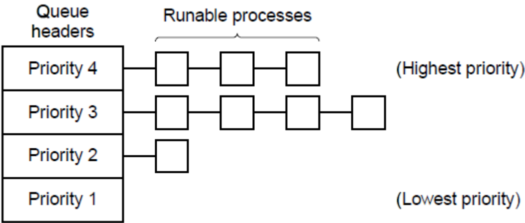
图2-23 一个有四类优先级的调度算法。
