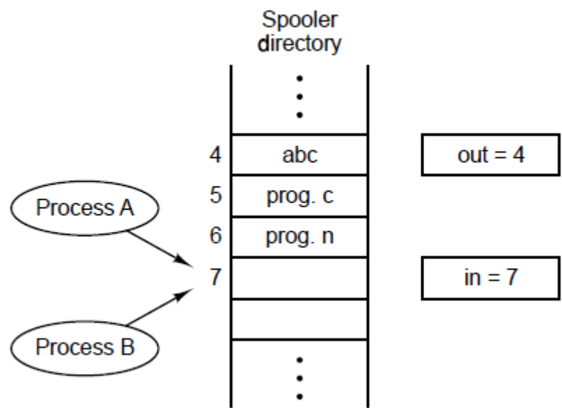
图2-7 两个进程试图在同一时刻访问共享内存。
