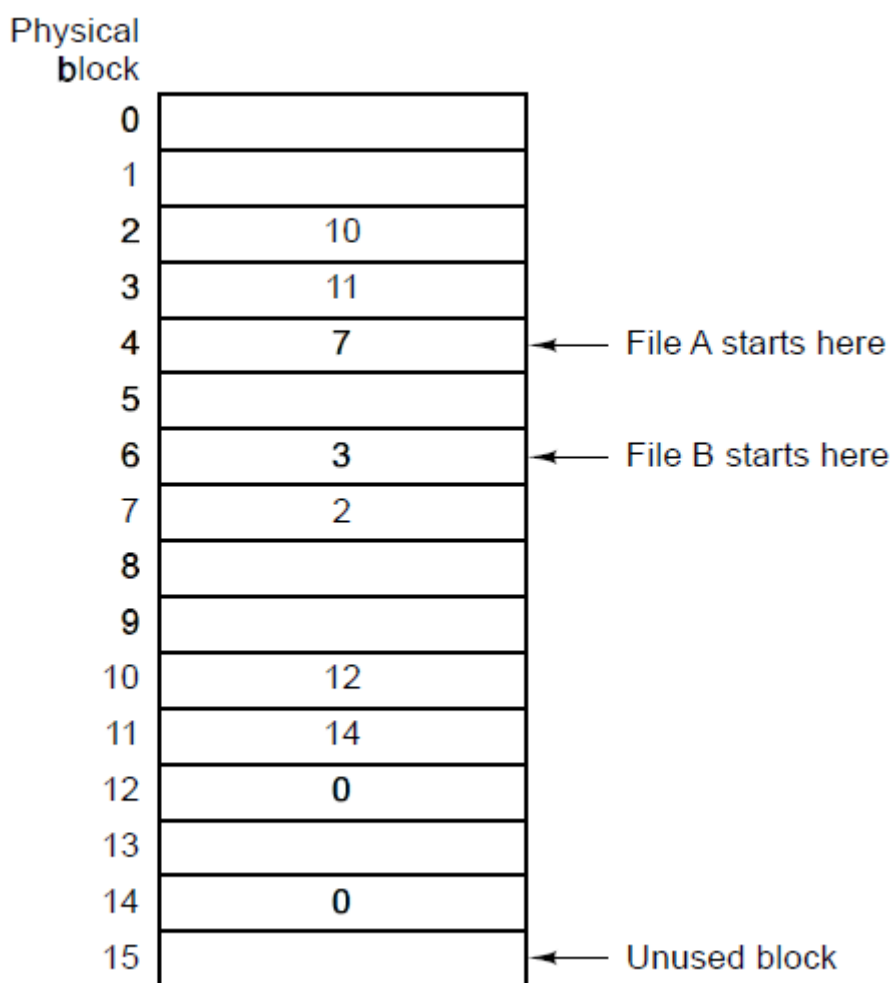
图5-9 使用内存表的链接表分配。
