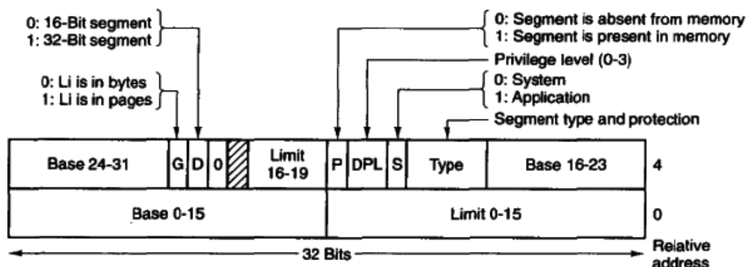
图4-28 奔腾的代码段描述符，数据段有轻微的差别。
