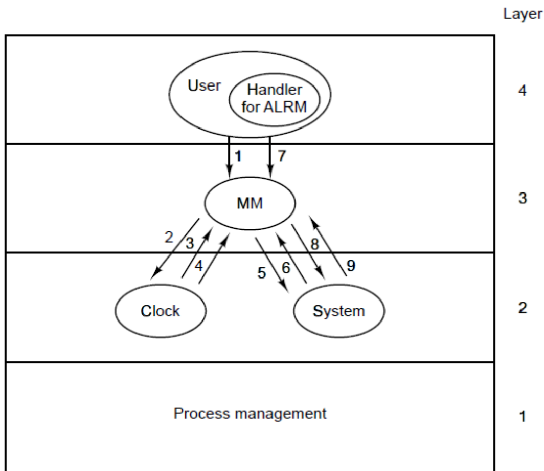
图4-45 与计时器有关的消息。其中最重要的有：(1)用户执行ALARM。(4)时间到信号被发出。(7)处理过程结束，调用SIGRETURN。详见文中描述。
