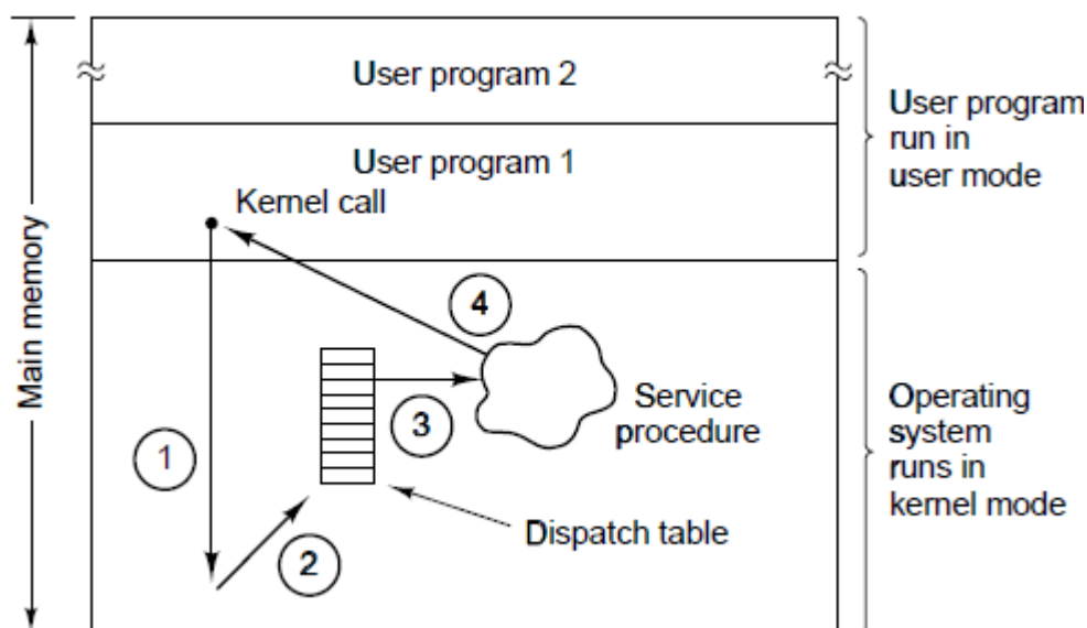
图 1-16 系统调用的操作过程：(1)用户程序陷入核心 (2)操作系统确定所请求的服务编号 (3)操作系统调用服务过程 (4)控制返回到用户程序
