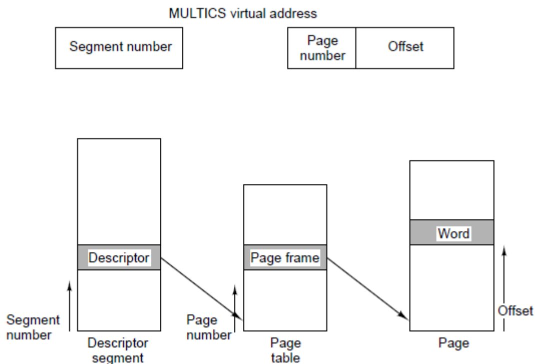
图4-25 两部分组成的MULTICS地址到主存地址的转换。
