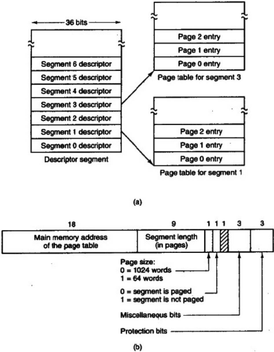
图4-23 MULTICS的虚拟存储器。(a)描述符段指向页表。(b)一个段描述符，其中的数字是各个域的长度 每个段都是一个普通的虚地址空间，用与本章前面讨论过的不分段的页式存储器相同的方式进行分页。一般的页面大小是1024字节（尽管有一些MULTICS自己使用的段不分页或以64字节为单位进行分页以节省存储器）。 一个MULTICS的地址有两部分构成：段和段内地址。段内地址又进一步分为页号和页内的内存字，如图4-24所示。在进行内存访问时，执行下面的算法。 1. 根据段号找到段描述符。 2. 检查该段的页表是否在内存中，如果在就找到它的位置，如果不在就发出一个段故障。如果访问违反了段的保护要求就发出一个故障（陷入）。 3. 检查所请求虚页的页表项，如果页面不再内存中则发出一个页面故障，如果在内存
