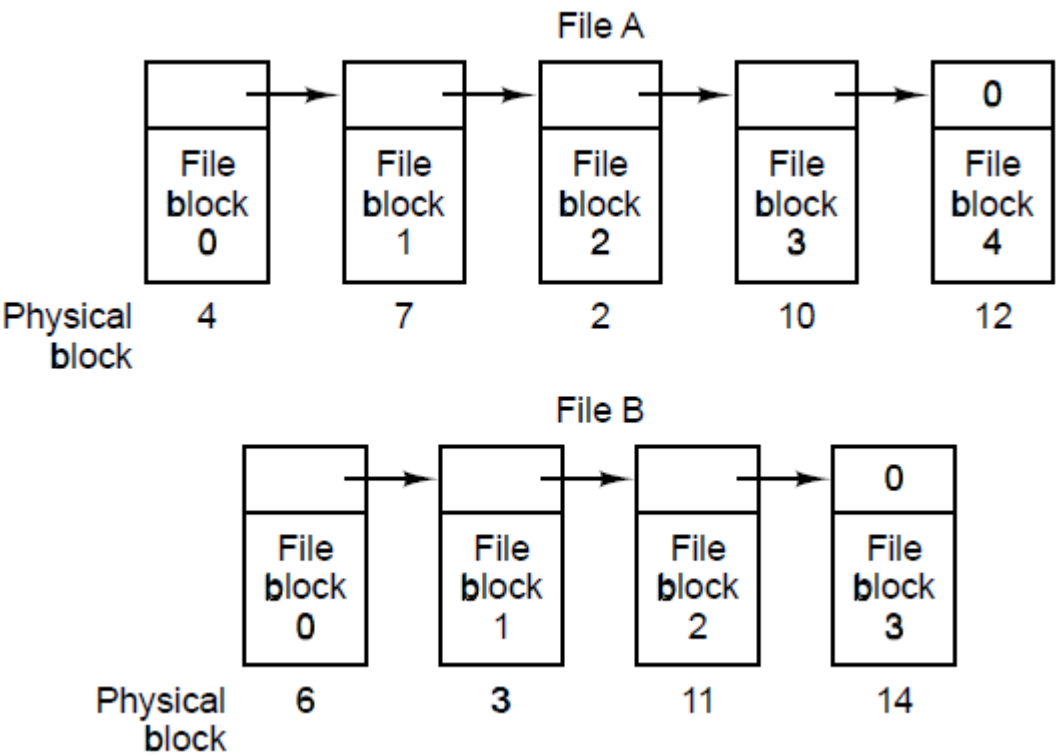
图5-8 按磁盘块链接表来存储文件。
