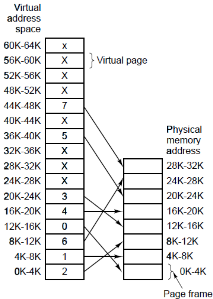
图4-8 虚地址与物理内存地址之间的关系由页表给出。
