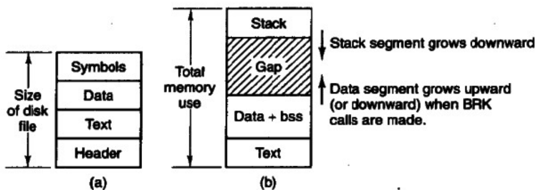
图4-33 (a)一个保存在磁盘文件中的程序。(b)一个进程的内部内存布局。在两图中最低的磁盘或内存地址都是在底端，最高的地址都是在顶端。
