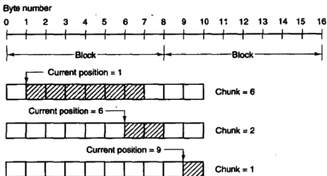
图5-39 三个例子表明在10字节文件中如何决定第一个小块的长度，块大小为8个字节，请求的字节数为6，小块用阴影显示。
