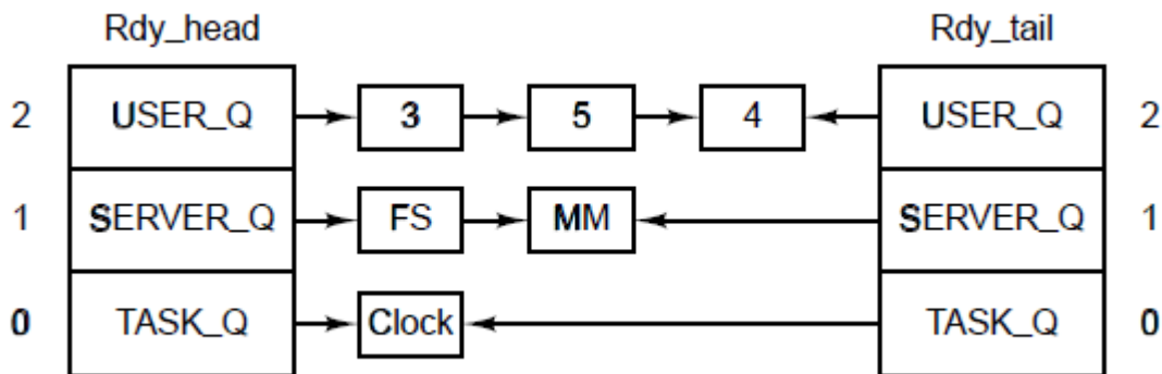
图 2-36 调度程序维护三个队列，每个优先级对应一个。
