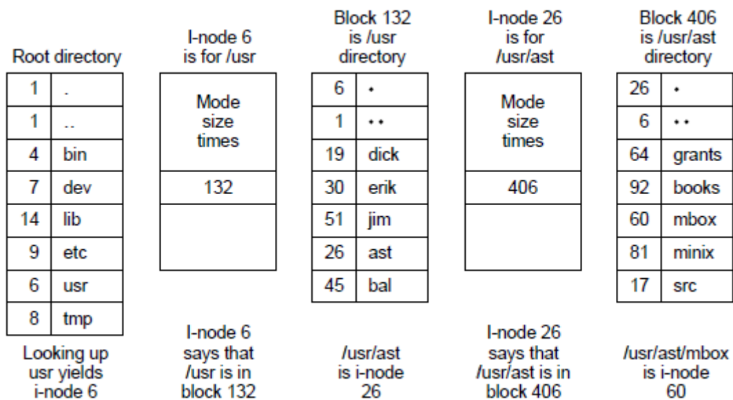
图5-14 查找 /usr/ast/mbox 的过程。
