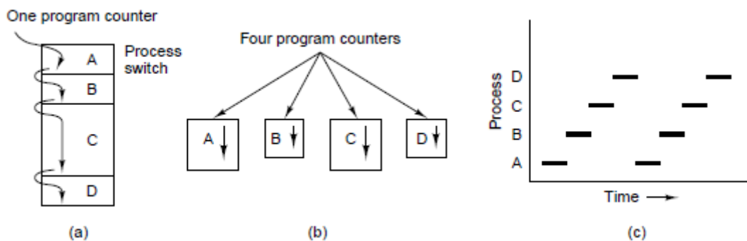
图2-1 (a) 多道程序中的四道程序。(b) 四个独立顺序进程的概念模型。(c) 在任意时刻仅有一个程序活跃。
