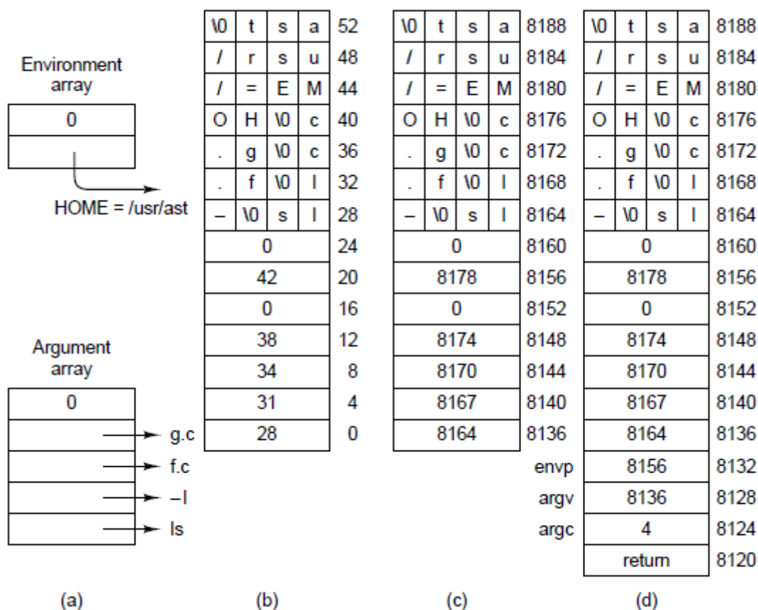
图4-39 (a)传给execve的数组 (b)execve构造的栈 (c)经内存管理器重新定位后的栈 (d)在main开始运行时的栈。
