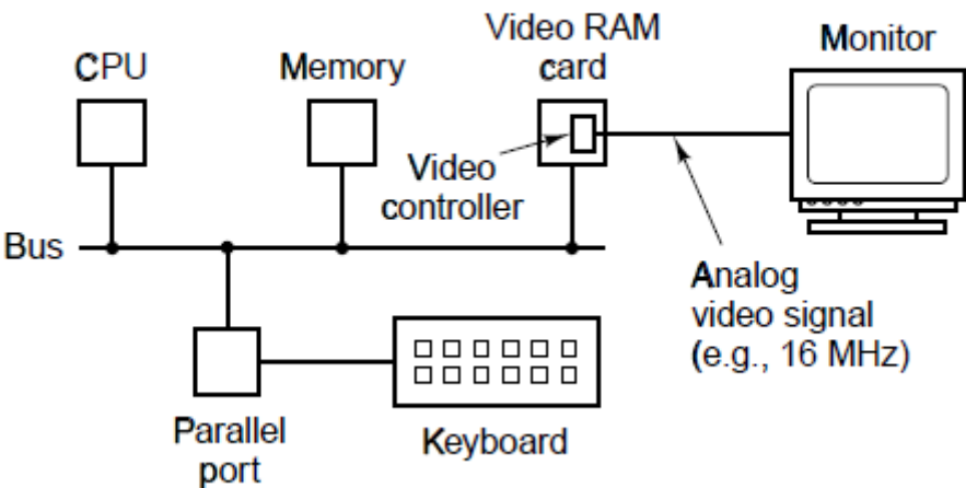
图 3-28 存储映像终端直接写入视频 RAM。
