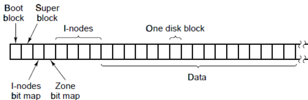
图5-28 最简单磁盘的磁盘布局，该磁盘为360K软盘，有128个i-节点，块大小为1K(即两个连续的512字节扇区作为一个块)。
