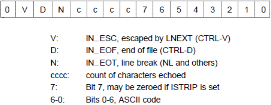
图 3-44 字符放入输入队列时字符码中的域。
