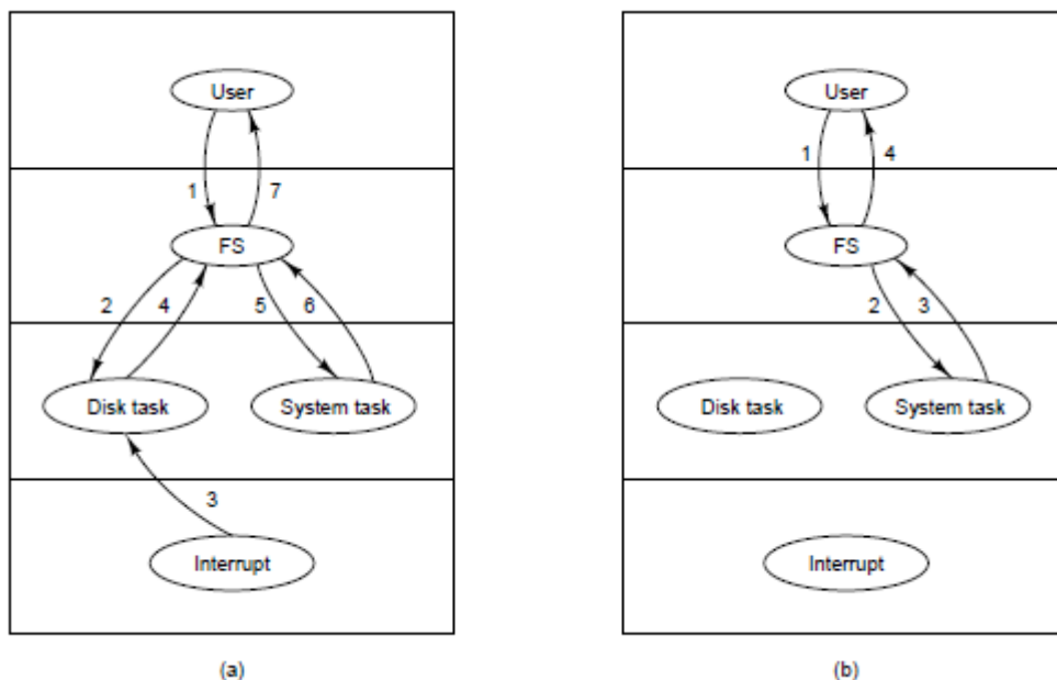
图 3-51 (a) 读一个块的最坏情况需要七条消息。(b) 读一个块的最好情况需要四条消息。
