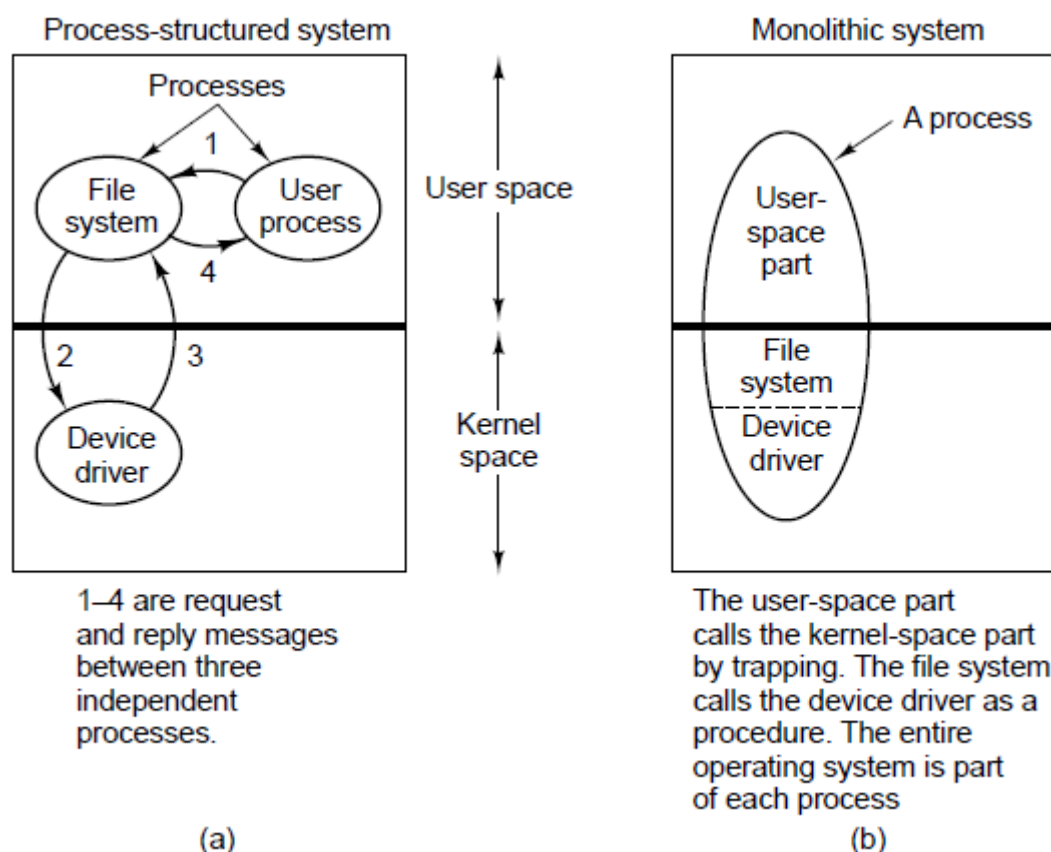
图 3-14 用户 — 系统通信的两种组织方式。
