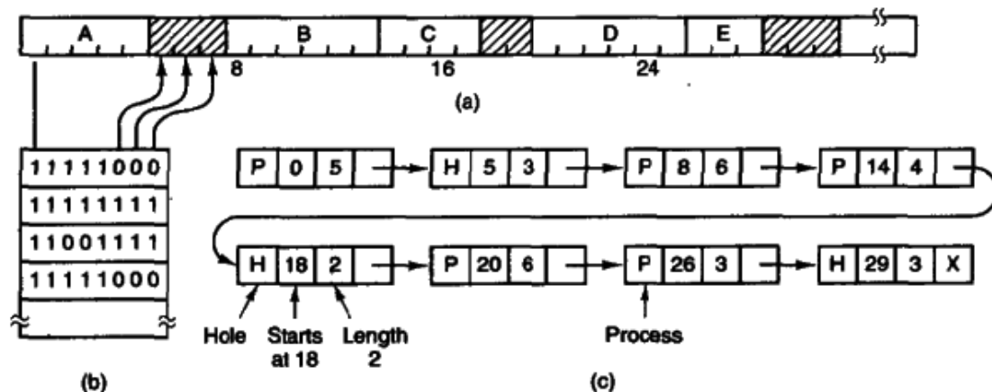
图4-5 (a)一段有五个进程和三个空洞的内存，刻度表示内存分配的单位，阴影表示空闲区域（在位图中用0表示）。(b)对应的位图。(c)用列表表示的同样的信息。
