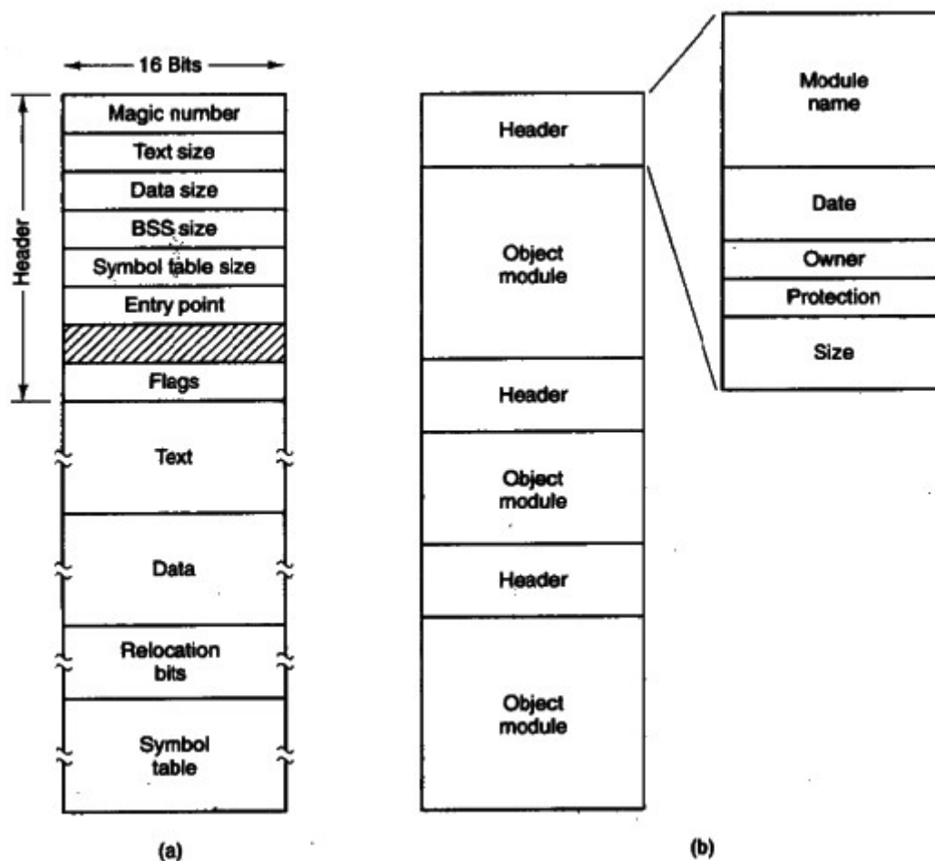
图5-3 (a)可执行文件。(b)存档文件。
