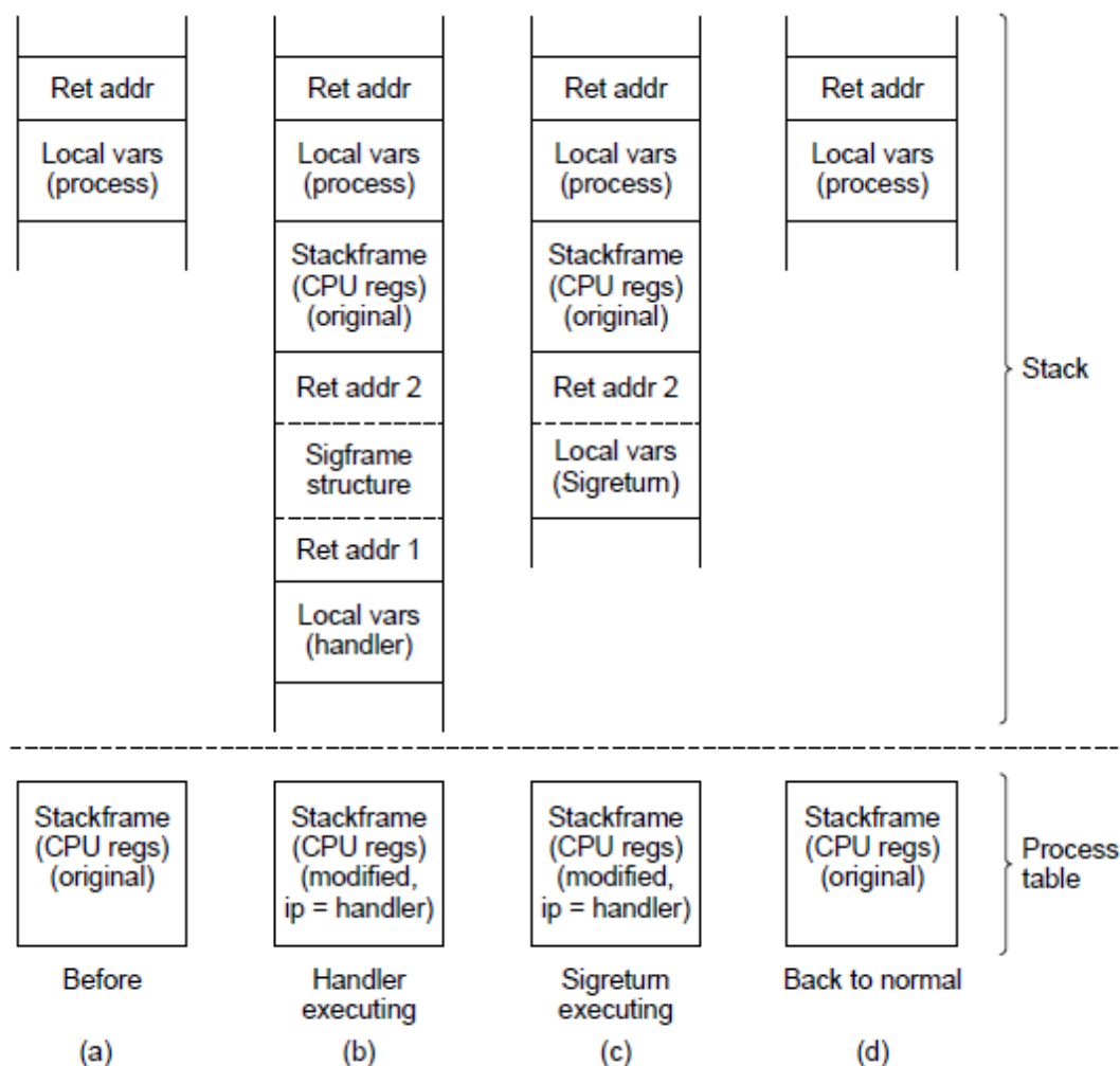
图 4-42 一个进程在处理信号不同阶段的栈（上面），和它在进程表中的栈框（下面）。(a)进程停止运行时的状态。(b)信号处理过程开始运行时的状态。(c)执行SIGRETURN时的状态。(d)SIGRETURN执行完之后的状态。
