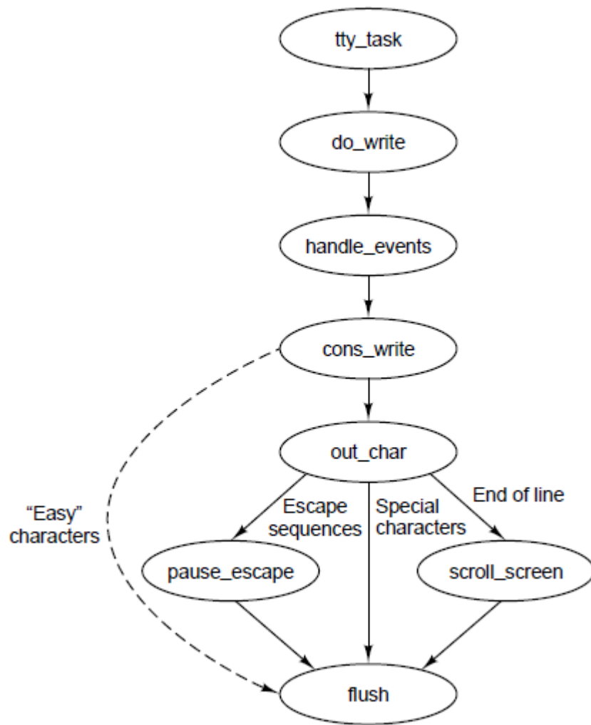
图 3-39 终端输出中使用的主要过程。虚线表示 cons_write 把字符直接拷贝到 ramqueue 。
