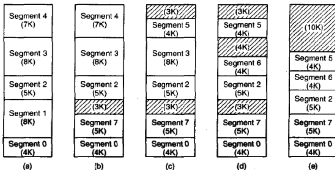
图4-22 (a)-(d)棋盘形碎片的形成。(e)通过紧缩消除棋盘形碎片。
