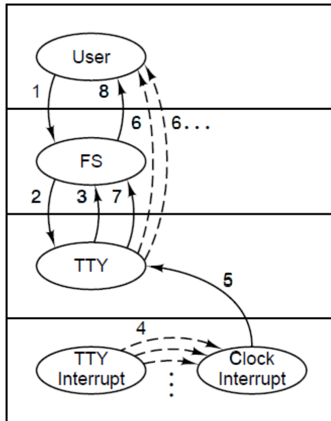
图 3-37 当还未输入字符时来自终端的读请求。FS 是文件系统，TTY 是终端任务。当输入字符时，终端的中断处理程序把输入字符排成一个队列，但是在这里由时钟中断处理程序唤醒 TTY。
