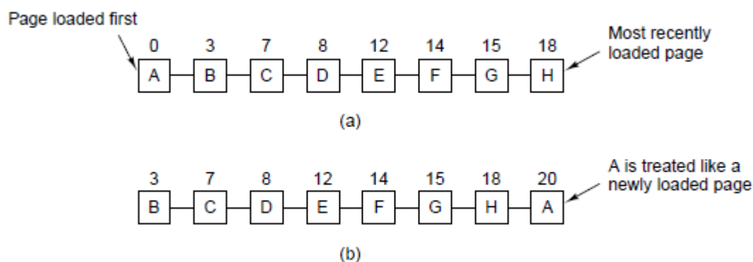
图4-13 第二次机会算法的操作。(a)页面按先进先出的顺序排列。(b)在时间20发生页面故障并且A的R位已经设置时的页面链。
