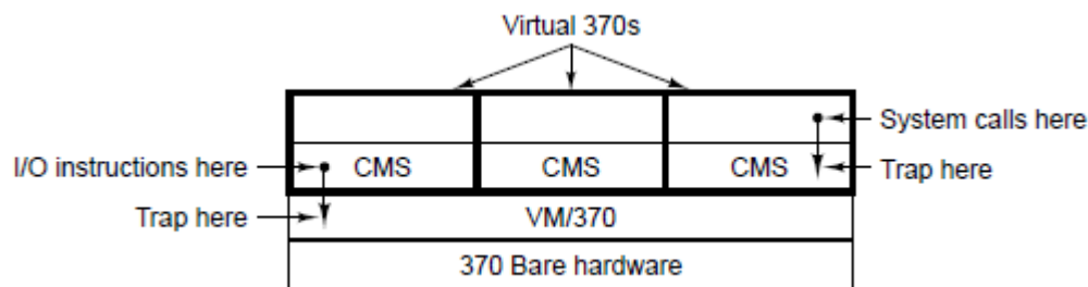
图 1-19 带CMS的VM/370结构。
