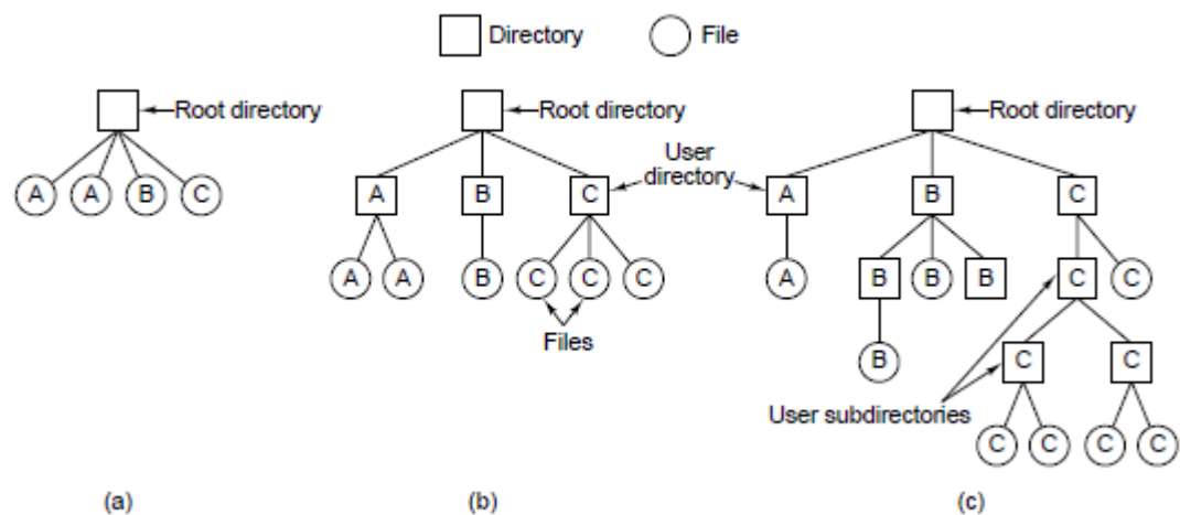
图5-6 三种文件系统设计。(a)所有用户共享一个目录。(b)每个用户拥有一个目录。(c)每个用户有一棵任意树。图中字母表示目录或文件拥有者。
