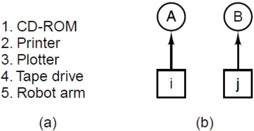
图 3-9 (a) 资源被赋予数字序号。(b) 一个资源图。
