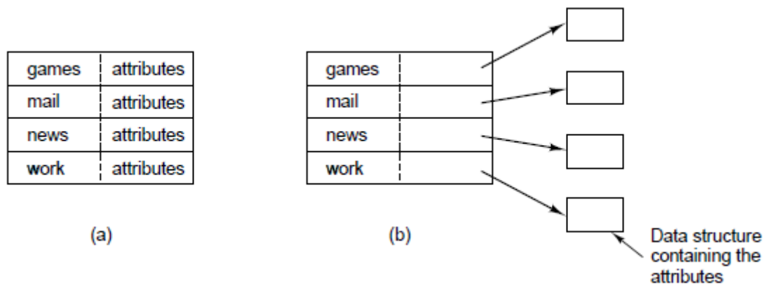
图5-5 (a)属性放在目录项中。(b)属性放在其他地方。
