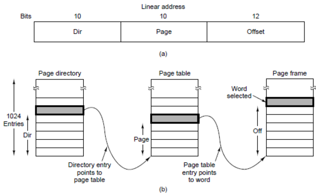
图4-30 线性地址到物理地址的映射。
