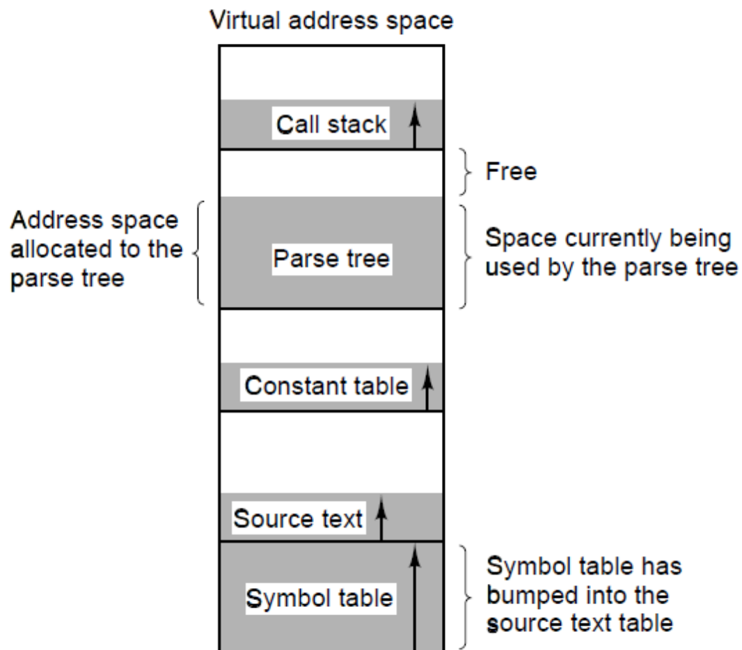
图4-19 在一维地址空间中，当有多个动态增长的表时，一个表可能会撞上另外一个。
