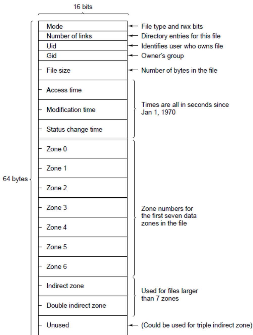
图5-30 MINIX i-节点。
