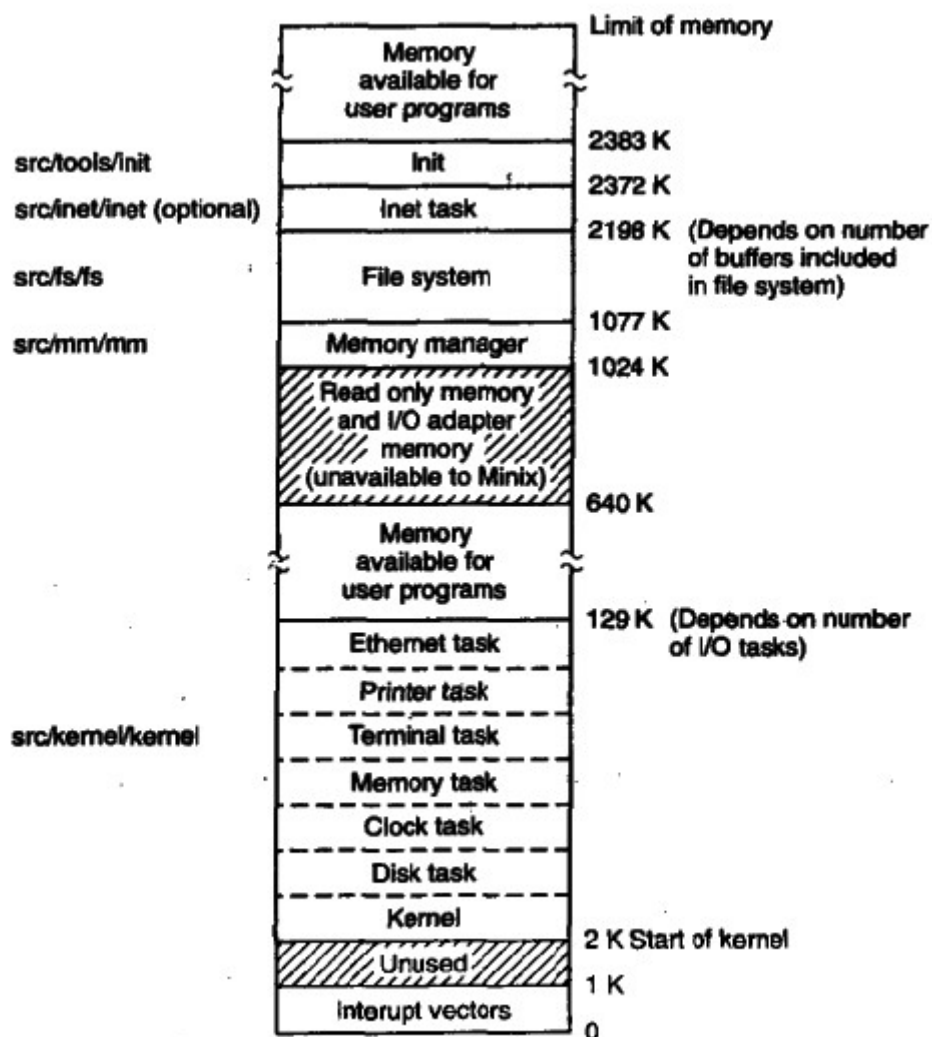
图 2-27 MINIX从磁盘装入内存之后的内存布局。四个单独编译并被链接的部分（若加上网络则为五部分）划分得很清楚。图中各部分的大小只是大概情况，具体则依赖于系统配置状况。
