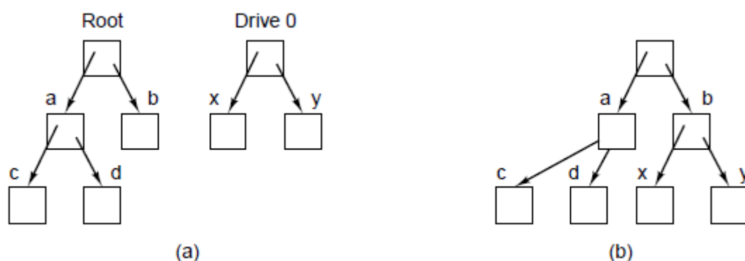
图 1-7 (a)在安装前，驱动器0中的文件不可访问。(b)安装后，驱动器0中的文件成为文件树的一部分。
