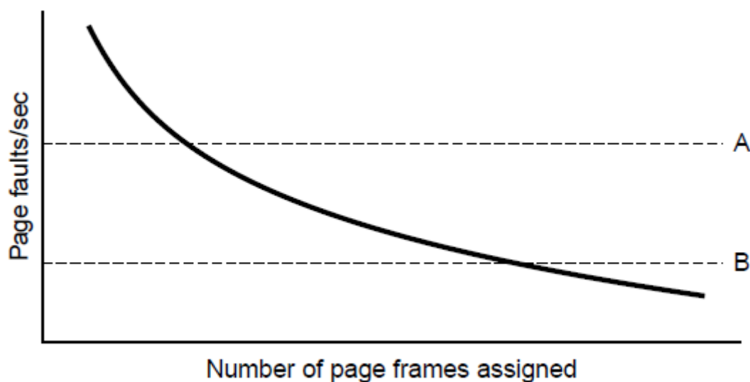
图4-18 页面故障率是分配的页框数的函数。
