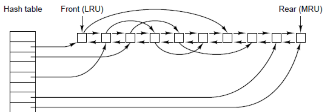
图5-31 块高速缓存使用的链接表。
