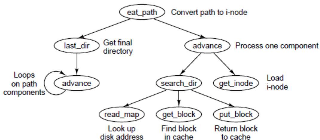
图5-42 用于查路径名的一些过程。
