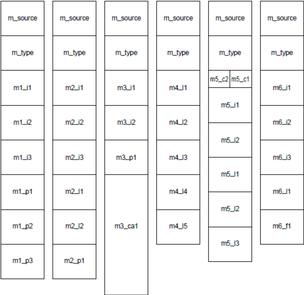
图 2-30 MINIX中使用的六种消息类型。消息元素的长度将随机器结构而变化；图中所示的是在32位指针机器，如Pentium (Pro)上的长度。
