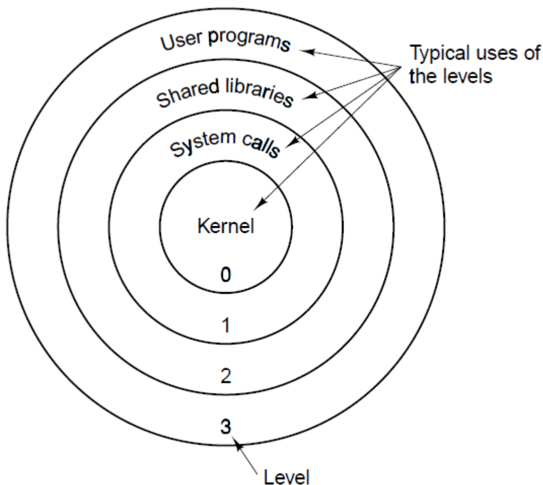
图4-31 奔腾中的保护。
