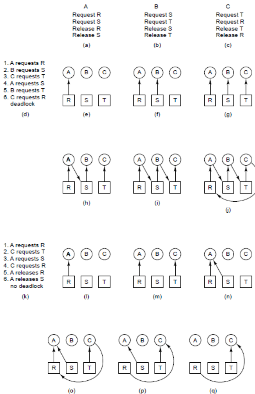
图 3-8 一个死锁如何发生和避免的例子。
