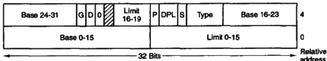
图 2-37 一个Intel处理器的段描述符格式。
