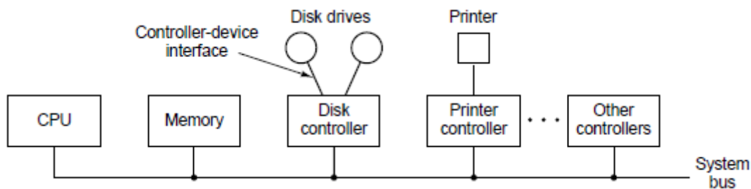
图 3-1 一个连接CPU、存储器、控制器和I/O设备的模型。
