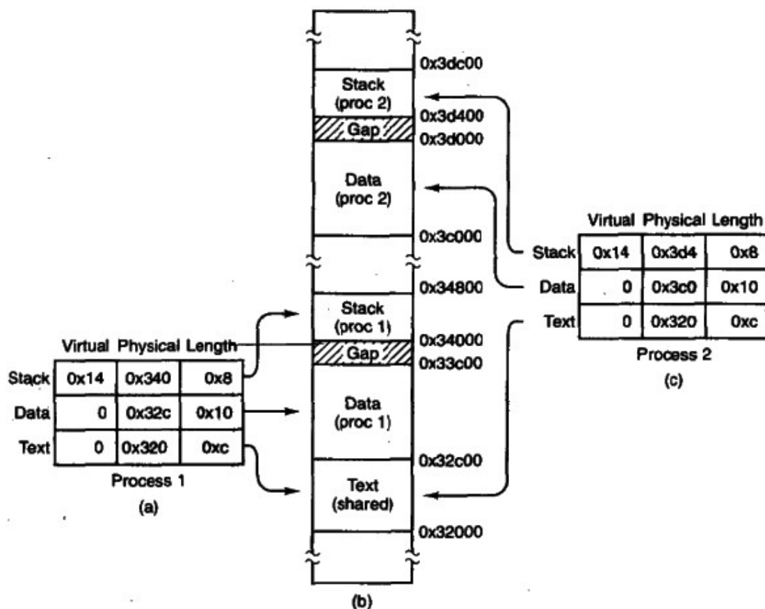
图4-36 (a)一个具有独立的I和D空间进程的内存映射，与上图相同。(b)第二个进程启动后的内存布局，他们通过共享正文执行相同的程序映像。(c)第二个进程的内存映射。
