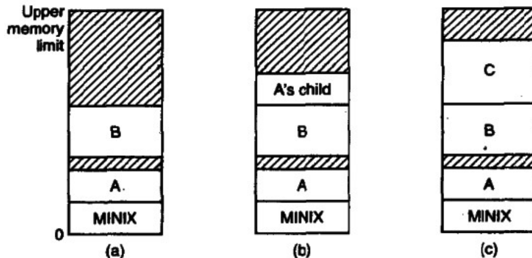
图4-32 内存分配。(a)原来的情况。(b)A执行FORK以后。(c)A的子进程执行了EXEC以后。阴影区域是未用内存。这个进程是一个普通的I和D结合的进程。
