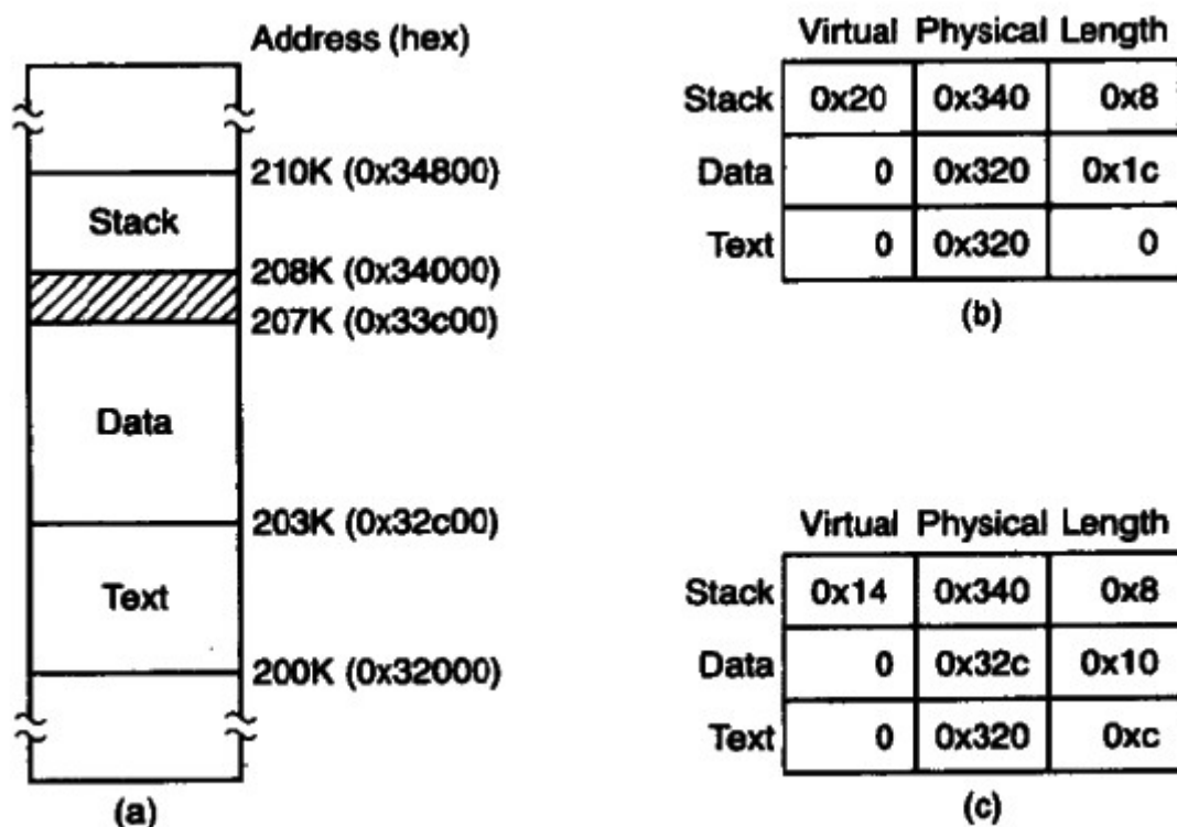
图4-35 (a)内存中的一个进程。(b)这个进程在I和D空间非独立时的内存表示。(c)I和D空间独立时的内存表示。
