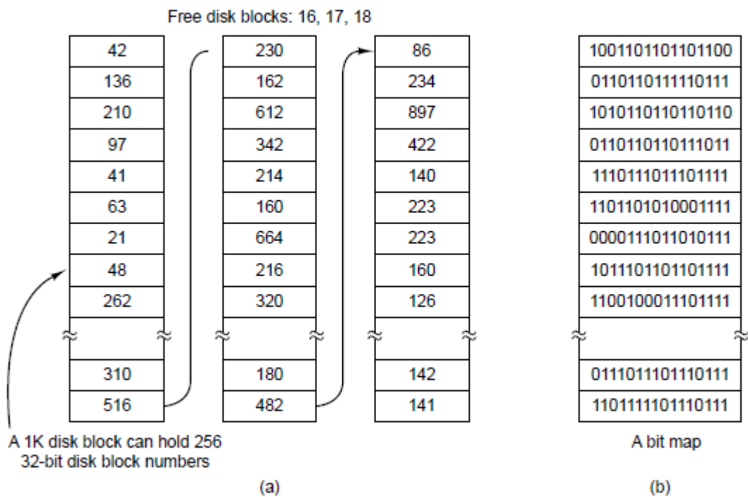
图5-16 (a)将空闲表存放在链接表中。(b)位图。
