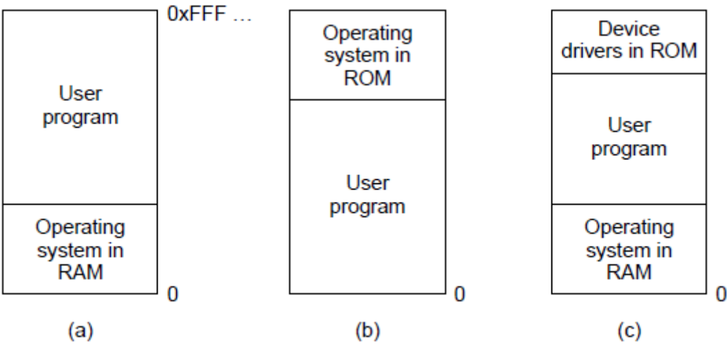
图4-1 在一个操作系统一个用户进程时三种简单的内存组织方法，其他方法也是存在的。
