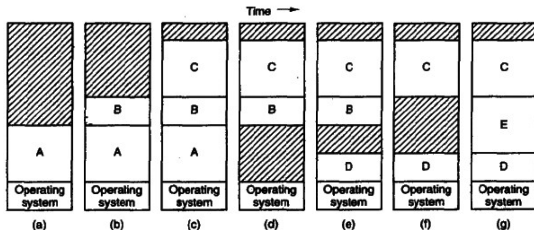
图4-3 内存分配情况随着进程进出内存而变化，阴影表示的区域是未使用的内存。
