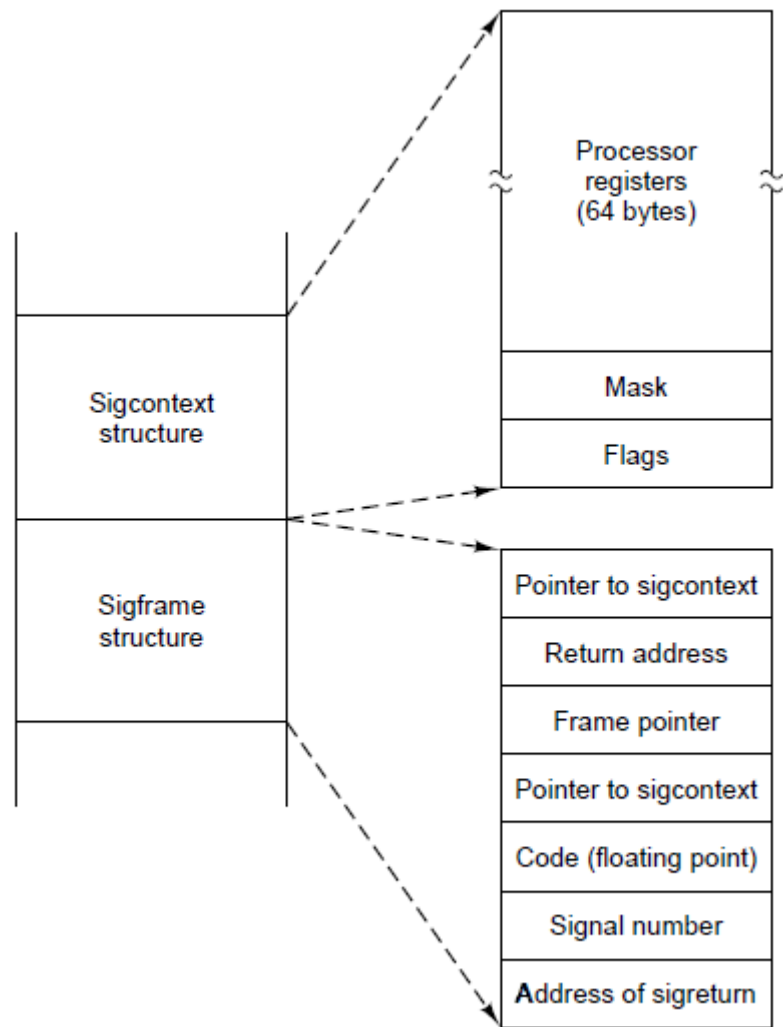
图4-46 为信号处理过程作准备而推入栈的sigcontext和sigframe结构。处理器的寄存器组是上下文切换时使用的栈框的一个拷贝。
