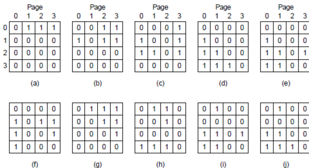
图4-15 使用矩阵的LRU算法。
