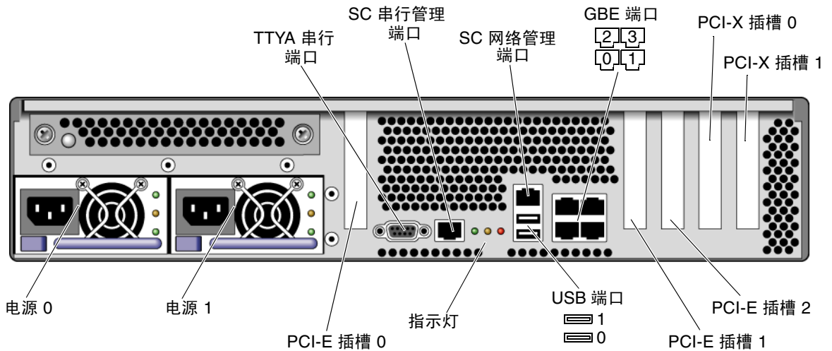
图 4 Sun Fire T2000 服务器后面板
