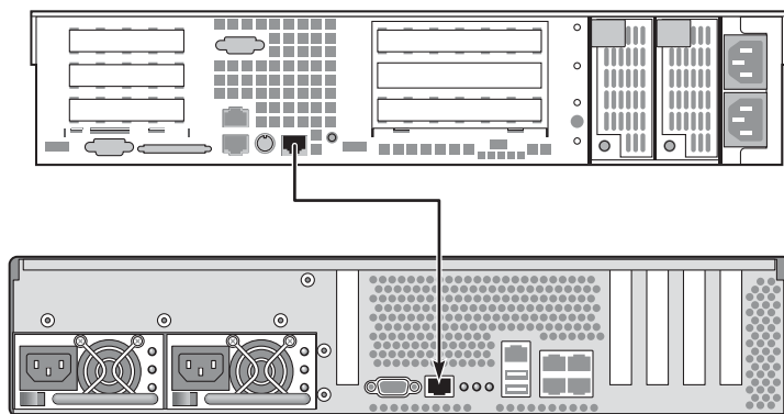
图 1-5 Sun Fire T2000 服务器与另一个 Sun 系统之间的 TIP 连接
