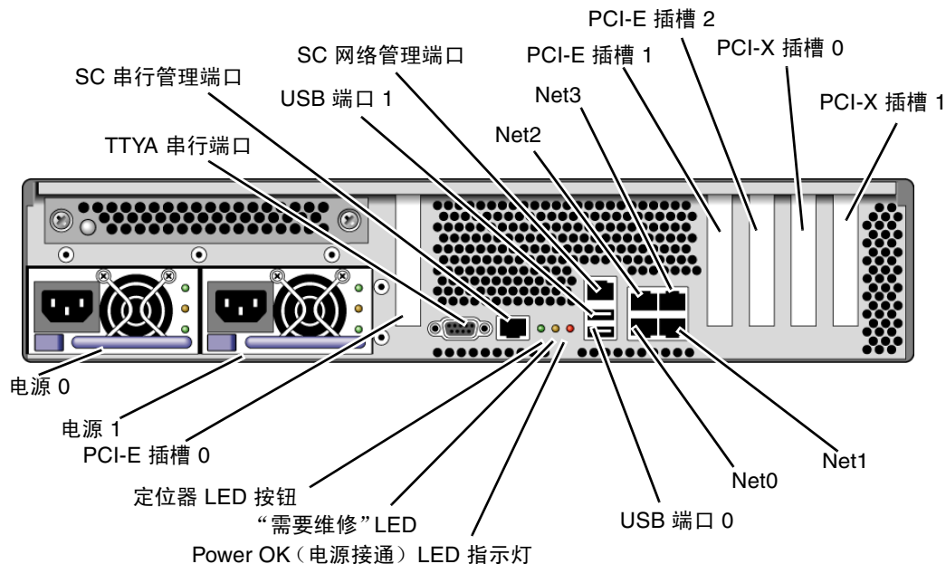
图 1-2 底盘后部 I/O 面板 — SC 串行管理端口是默认的控制台连接
