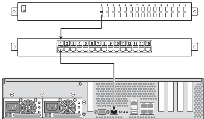
图 1-4 通过插线板连接终端服务器和 Sun Fire T2000 服务器
