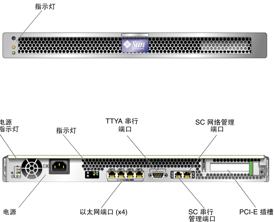
图 3 Sun Fire T1000 服务器的前后面板
