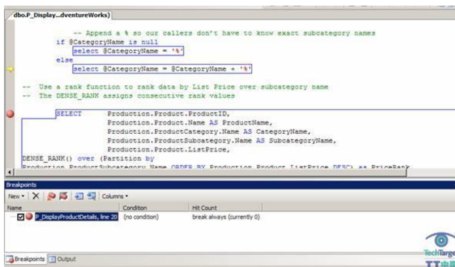
图 7：断点窗口
