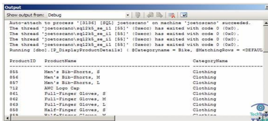
图 6: 输出窗口
