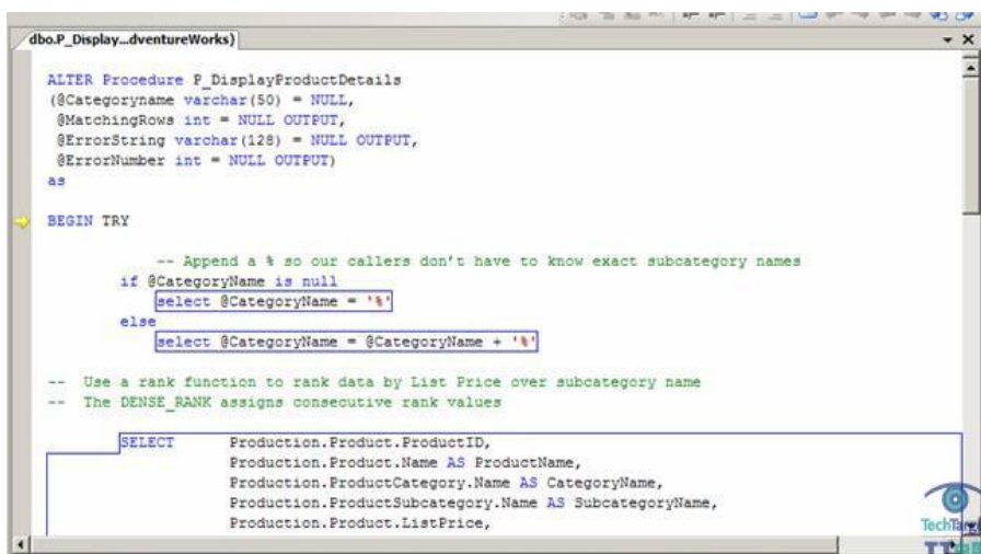
图 3：待执行代码
