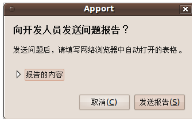
图 9.27 缺陷跟踪
