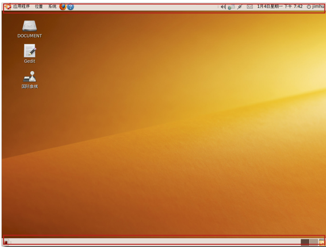
图 2.3 桌面面板
