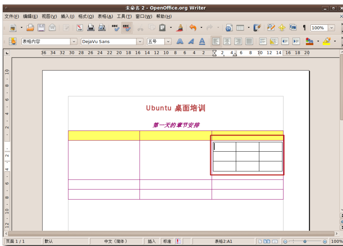
图 4.15 嵌套表格
