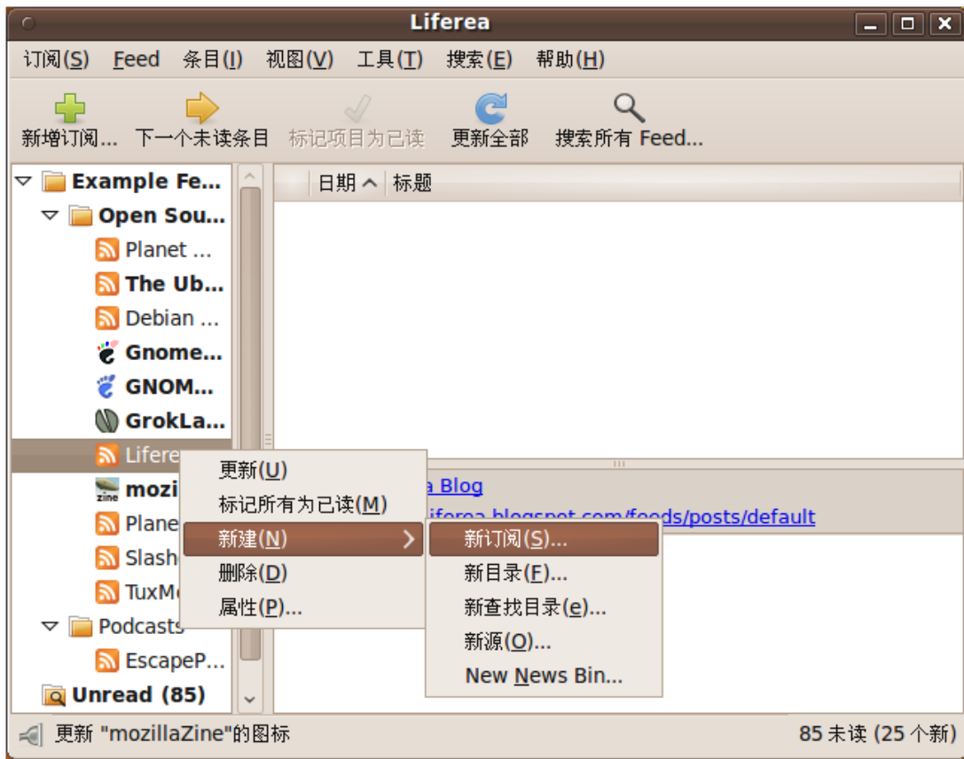
图 3.18 订阅 RSS
