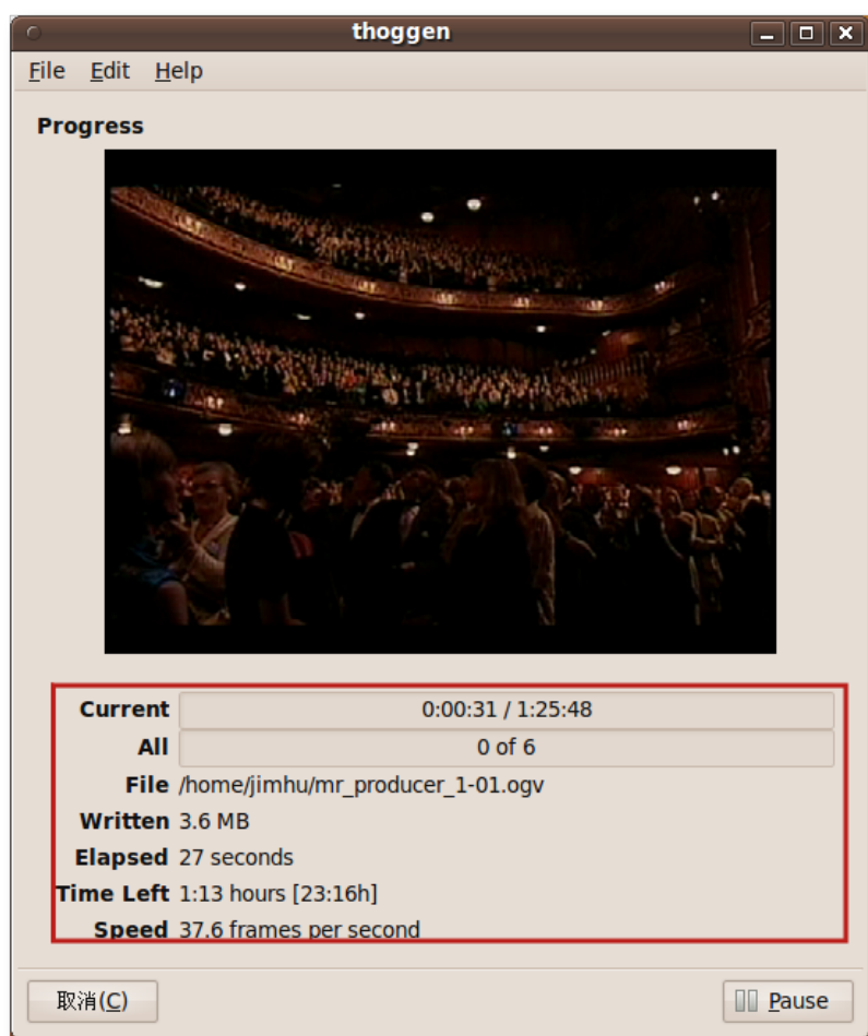
图 8.73 备份 DVD
