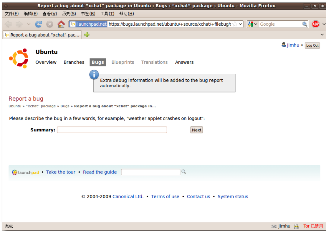
图 9.28 缺陷报告
