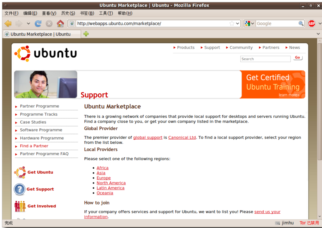
图 9.34 Canonical 市场
