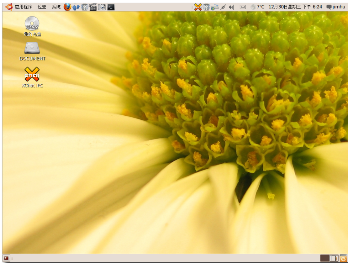
图 6.7 添加的墙纸
