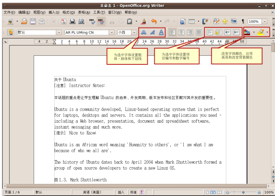
图 4.5 格式工具栏
