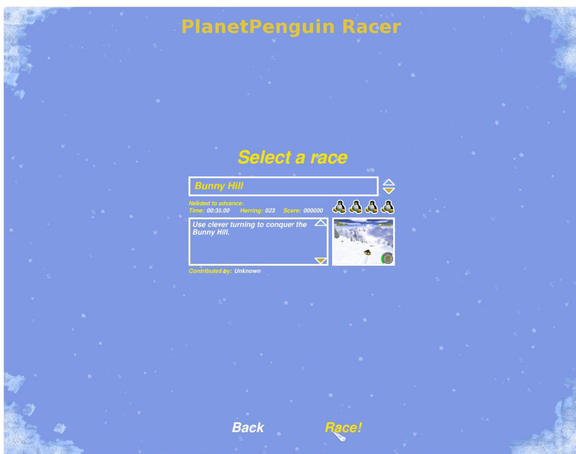
图 5.18 选择赛道
