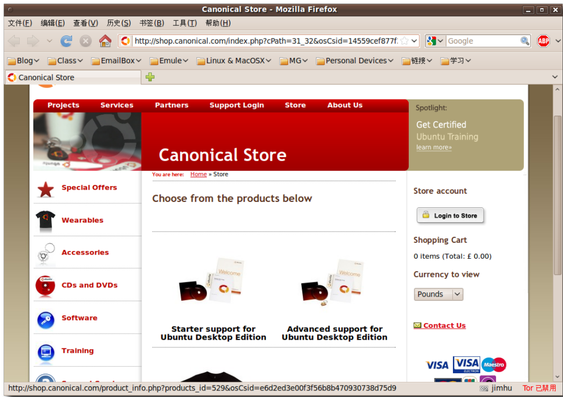
图 9.33 关于我们
