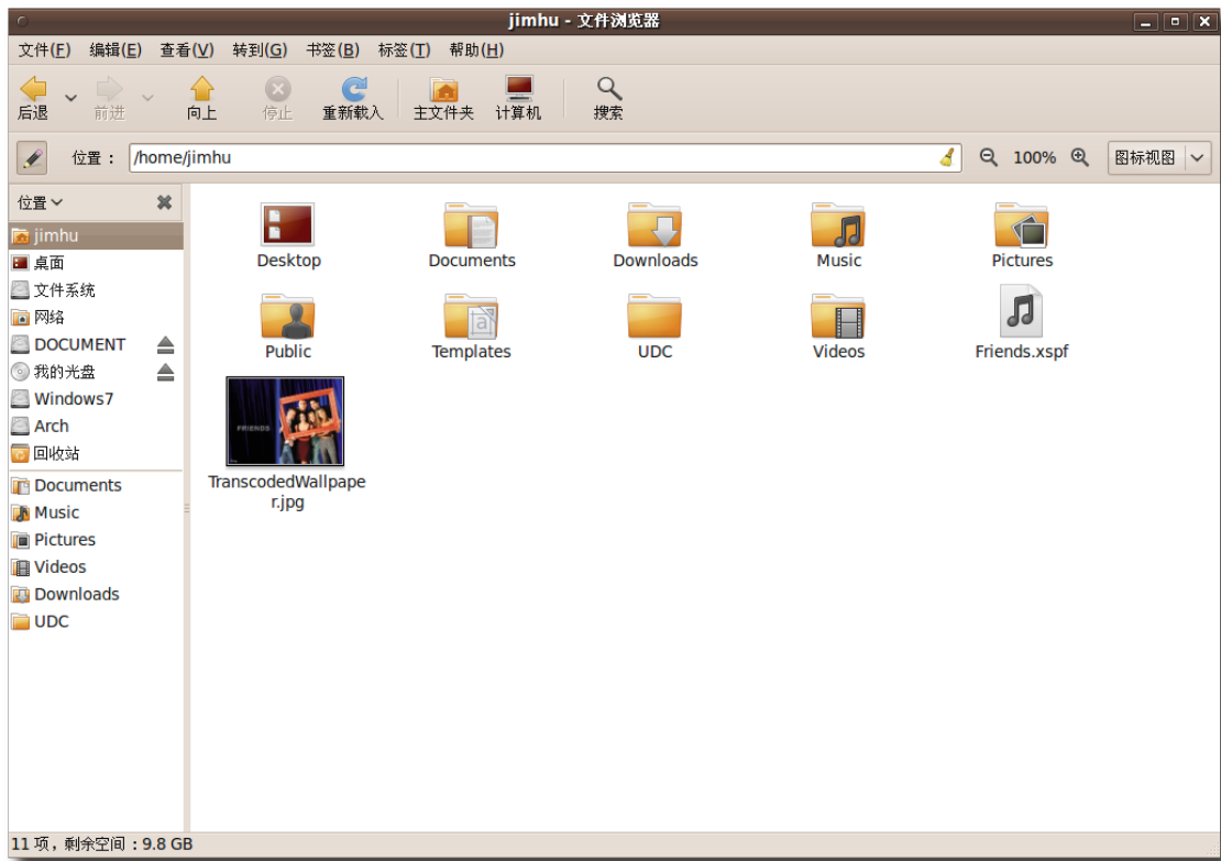
图 6.28 文件显示
