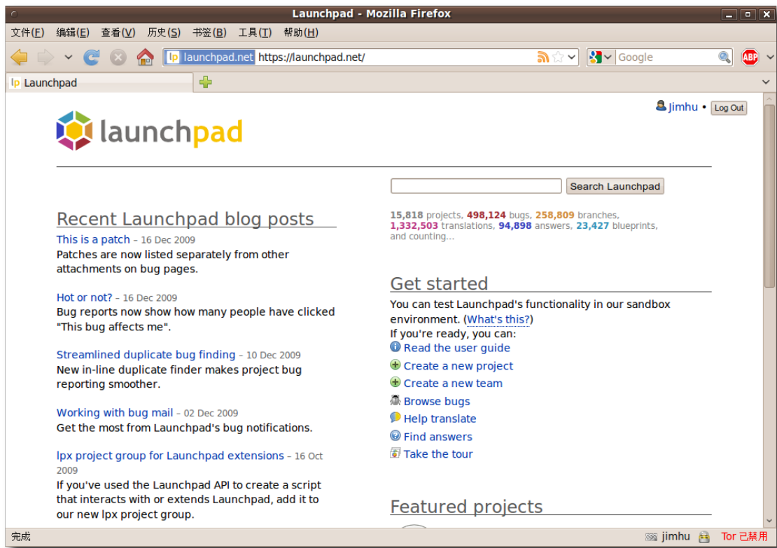
图 9.21 Launchpad
