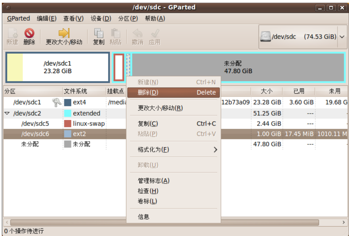
图 10.8 删除分区
