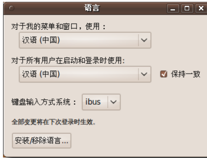
图 2.25 语言对话框
