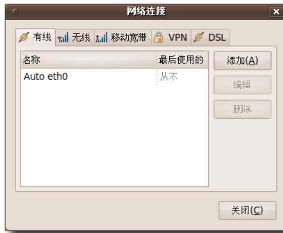
图 3.4 网络设置
