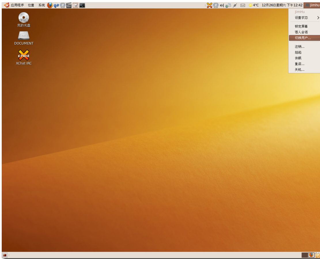
图 2.31 切换用户
