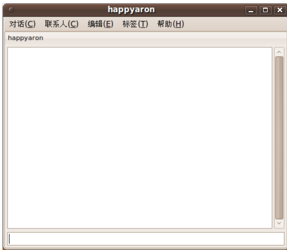
图 3.49 聊天窗口
