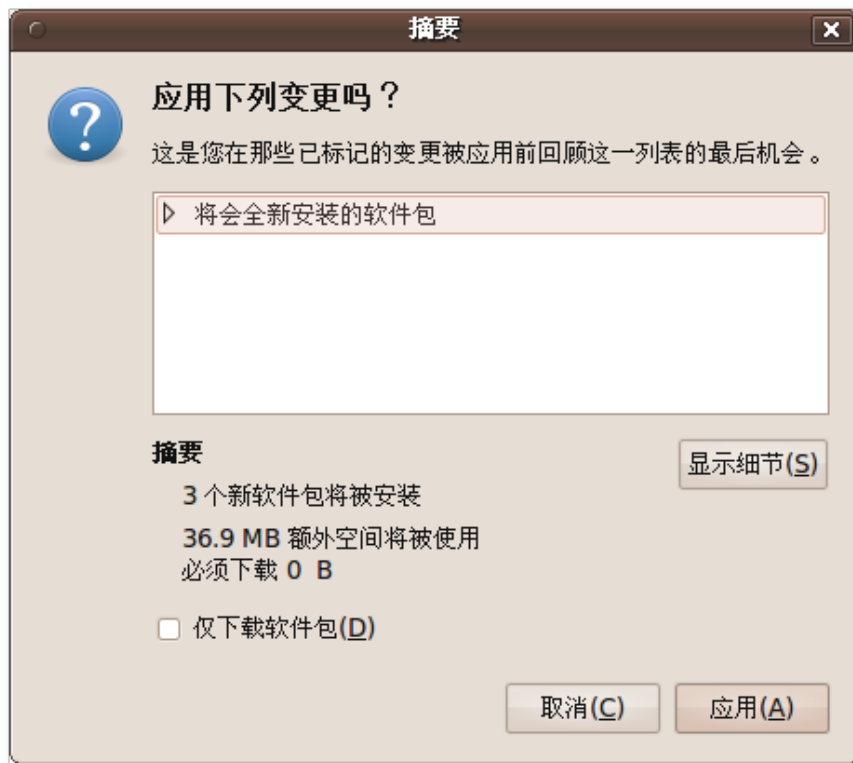
图 3.35 确认变更
