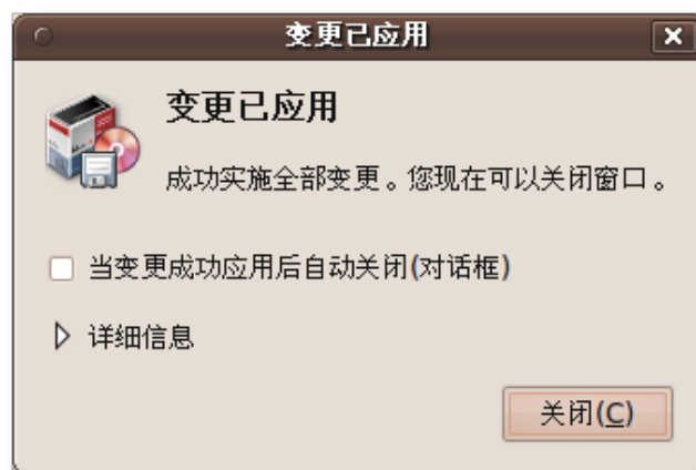
图 6.47 安装完成
