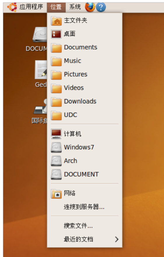
图 2.5 “位置”菜单
