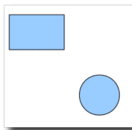
图 4.74 框架选定
