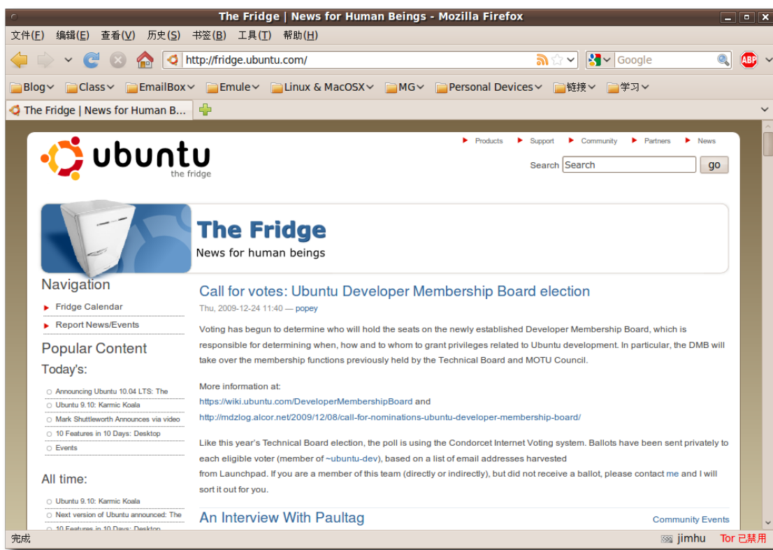
图 9.31 Fridge 新闻站
