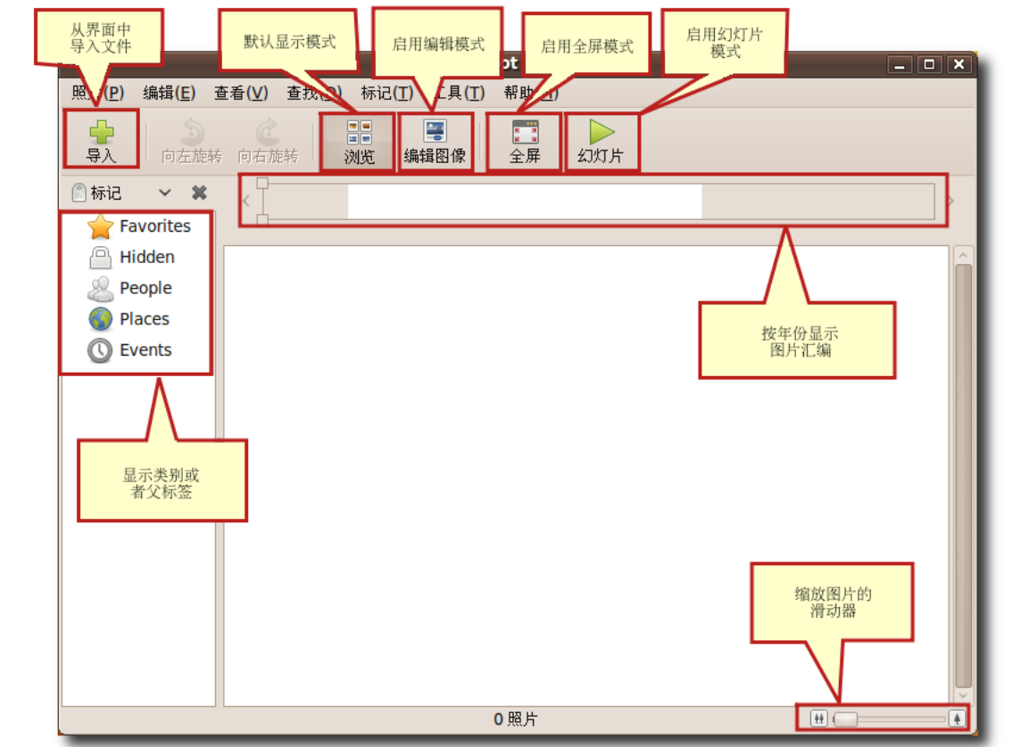
图 7.1 F-Spot 窗口
