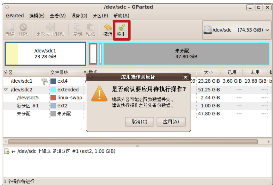
图 10.5 确认对话框
