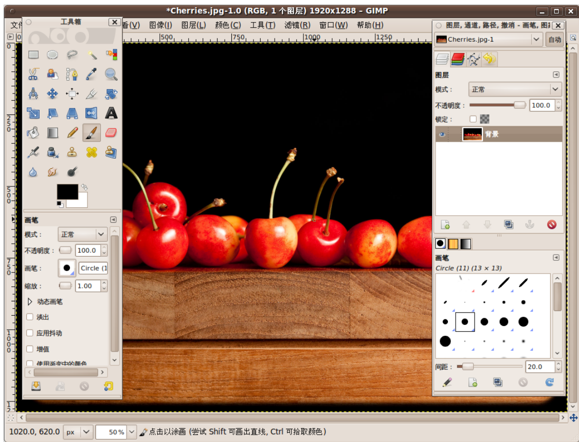
图 1.10 GIMP
