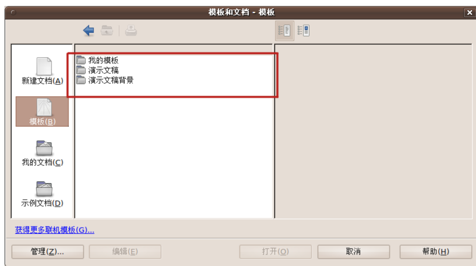
图 4.4 使用模板
