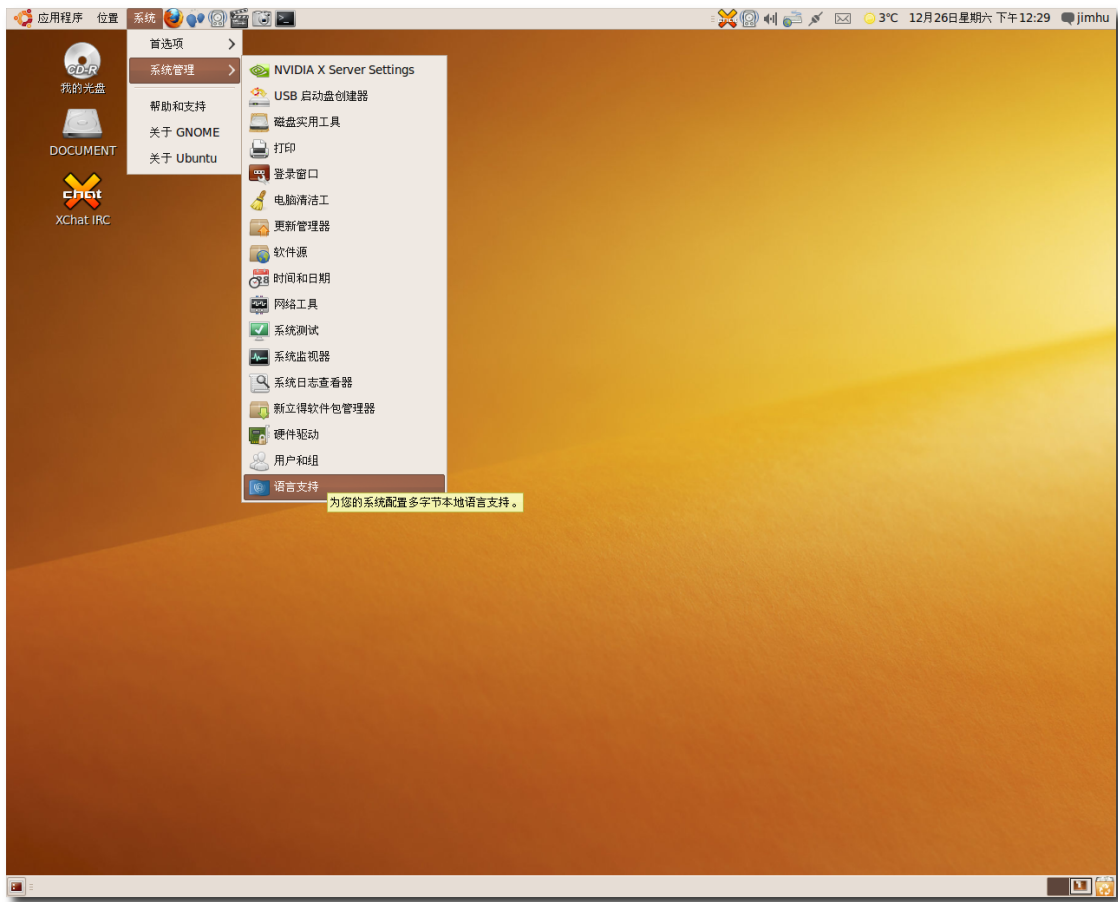
图 2.24 配置语言
