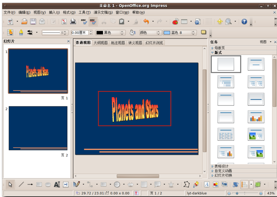
图 4.60 三维文本
