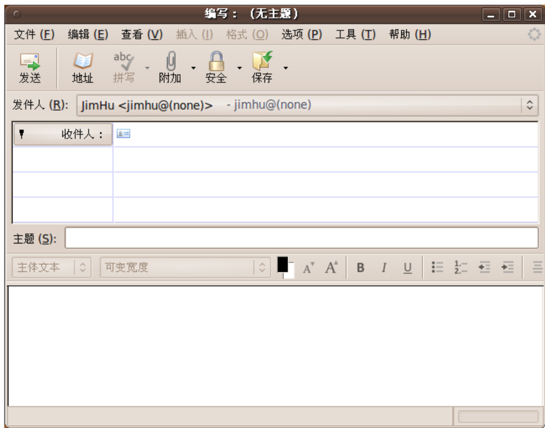
图 3.40 拼写检查器
